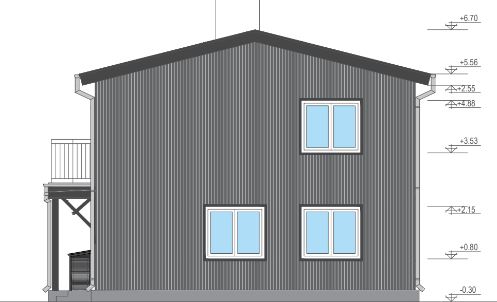
Vaade loodest M1:100
