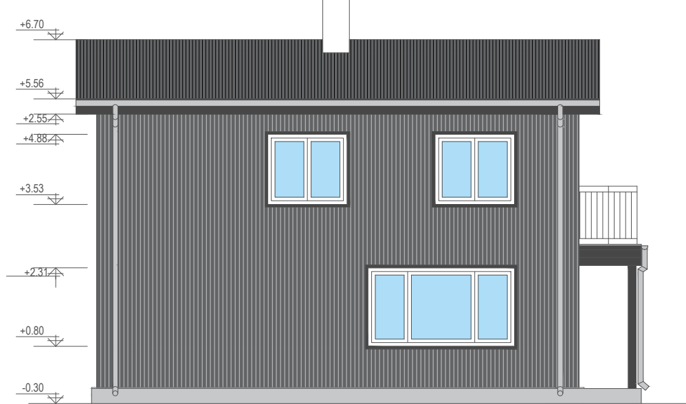
Vaade edelast M1:100
