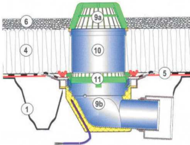
Joonis. Kaheastmeline küttegaabli ja kondensirõngaga ( 11 ) varustatud äravoolukaev.
