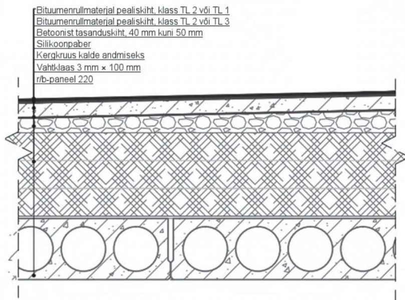
Joonis A.10 — Tavapärase bituumenrullmaterjaliga katus niisketele ruumidele.
