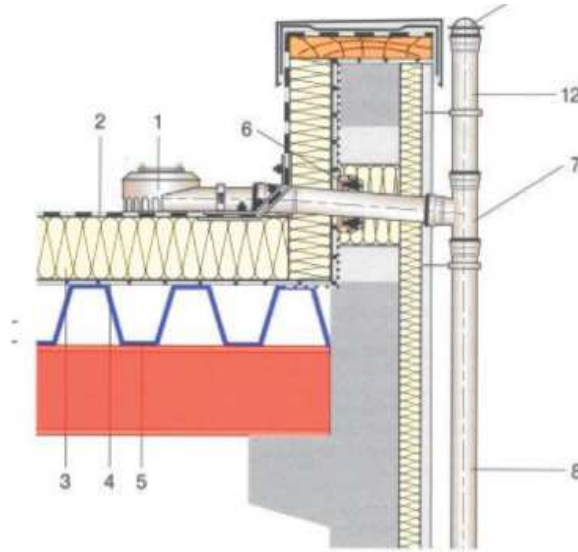
Foto Sülitil abil parapetti läbiv sisemise- ja välimise äravoolu kombinatsioon.
