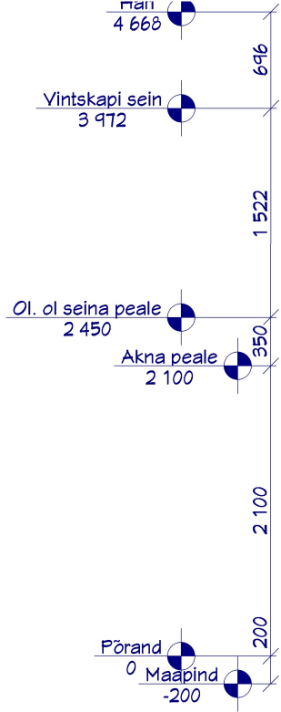
Vaade Idast
