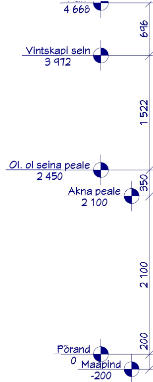
Vaade Põhjast
