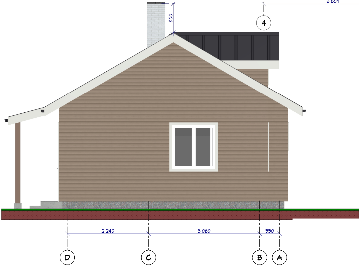
Vaade Idast
