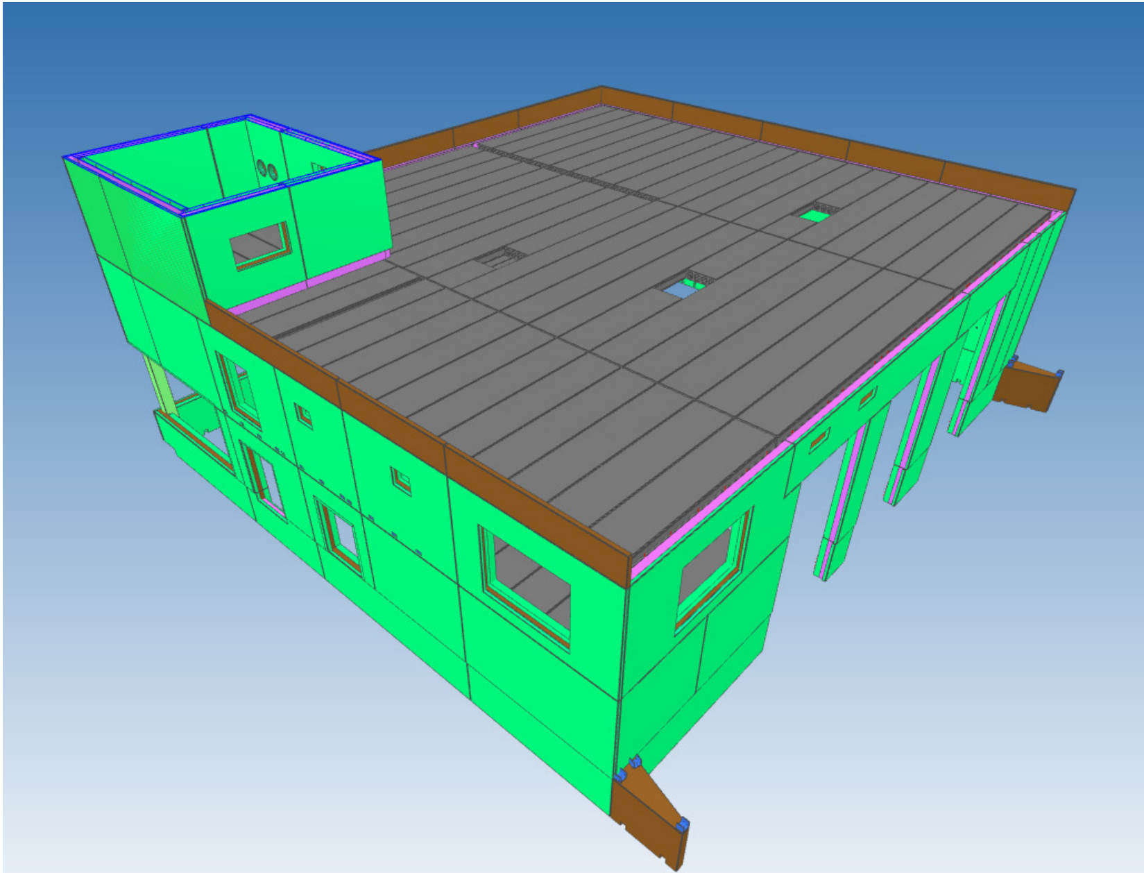
Parapetid ja 3.korruse seinalemendid - MONTAAŽ 6
