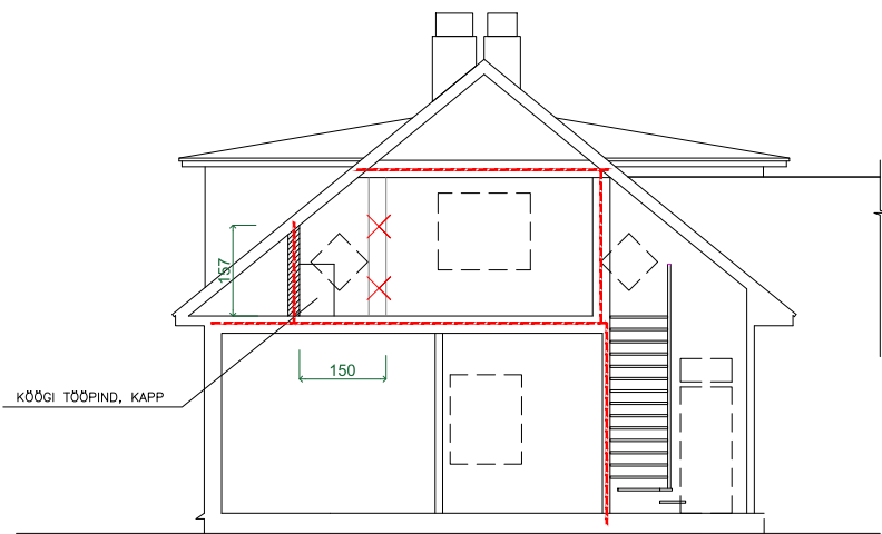
LÕIGE I-I
