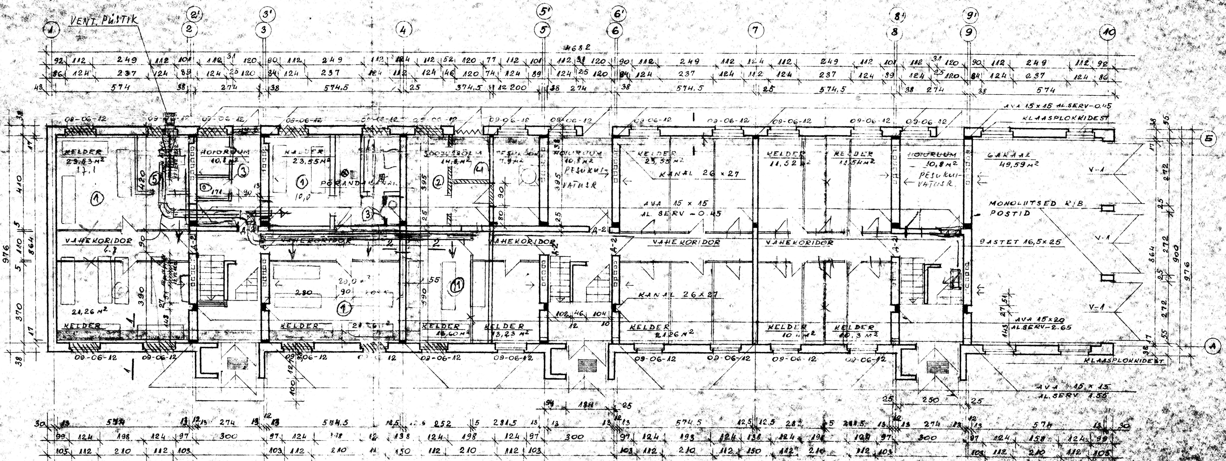
PÕRANDAALUSED KANALID
