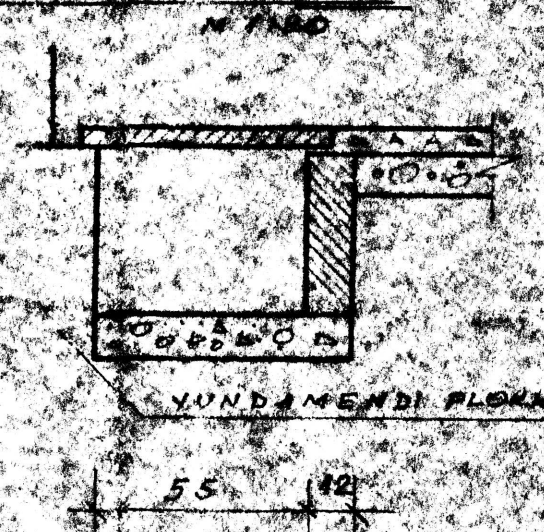
LÕIGE 2-2
