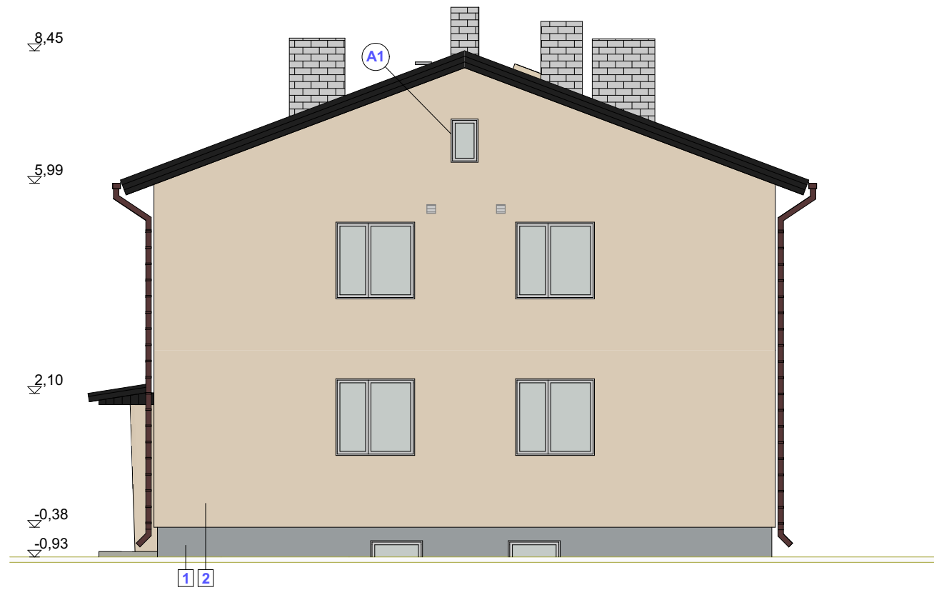
Vaade B
