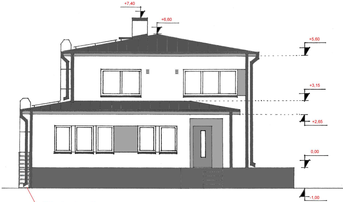
Vaade C
