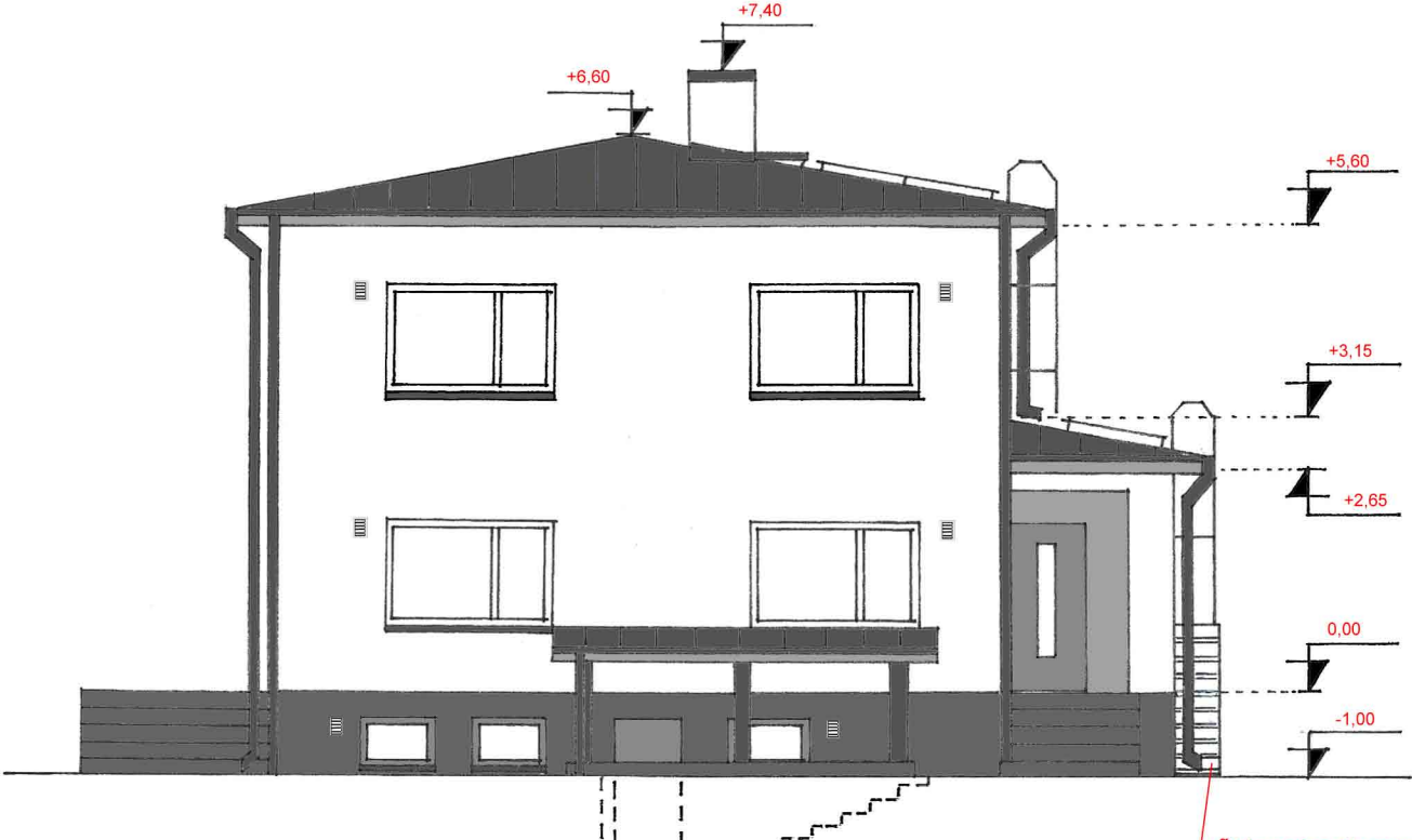
Vaade A
