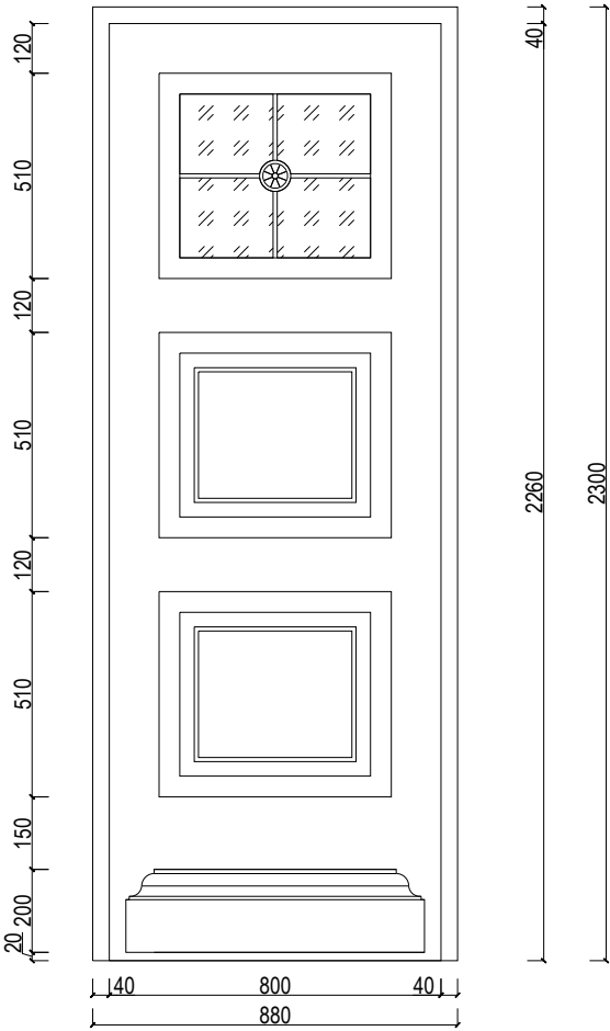
Välisuks VU-2
