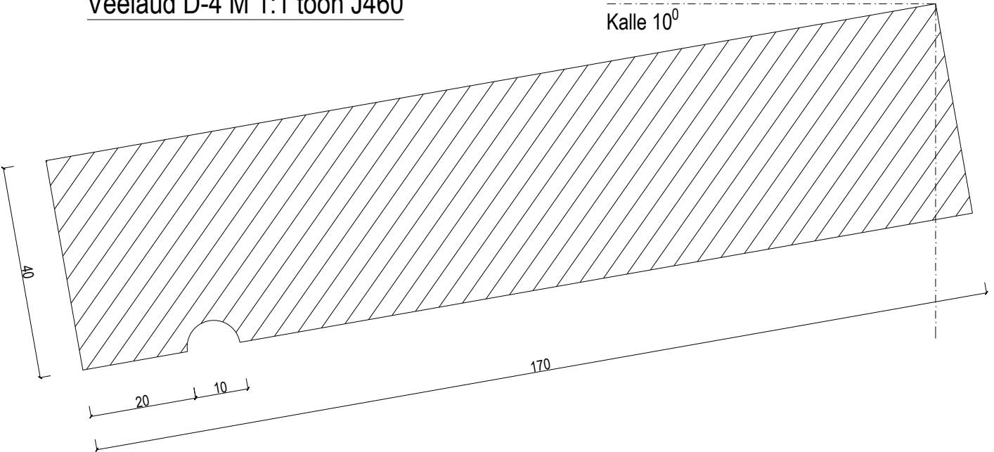
Veelaud D-4 M 1:1 toon J460
