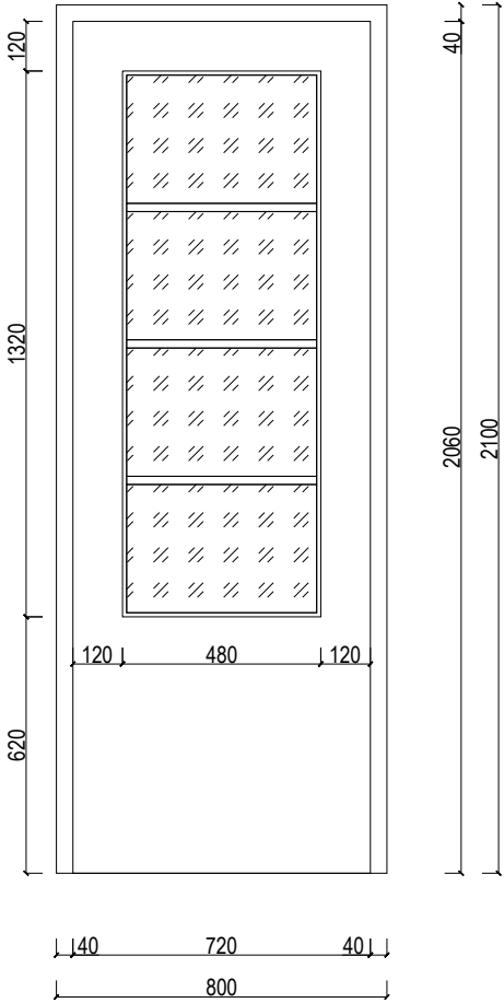
Välisuks VU-3
