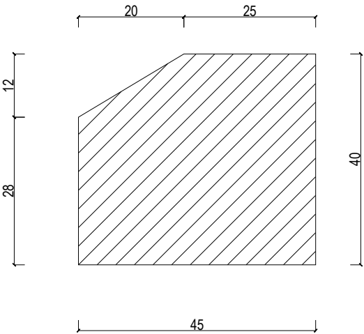
Aknaalune karniis D-9 M 1:1 toon F461
