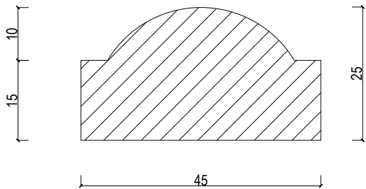
Akende ja uste piirdelaud D-6 M 1:1 toon F461
