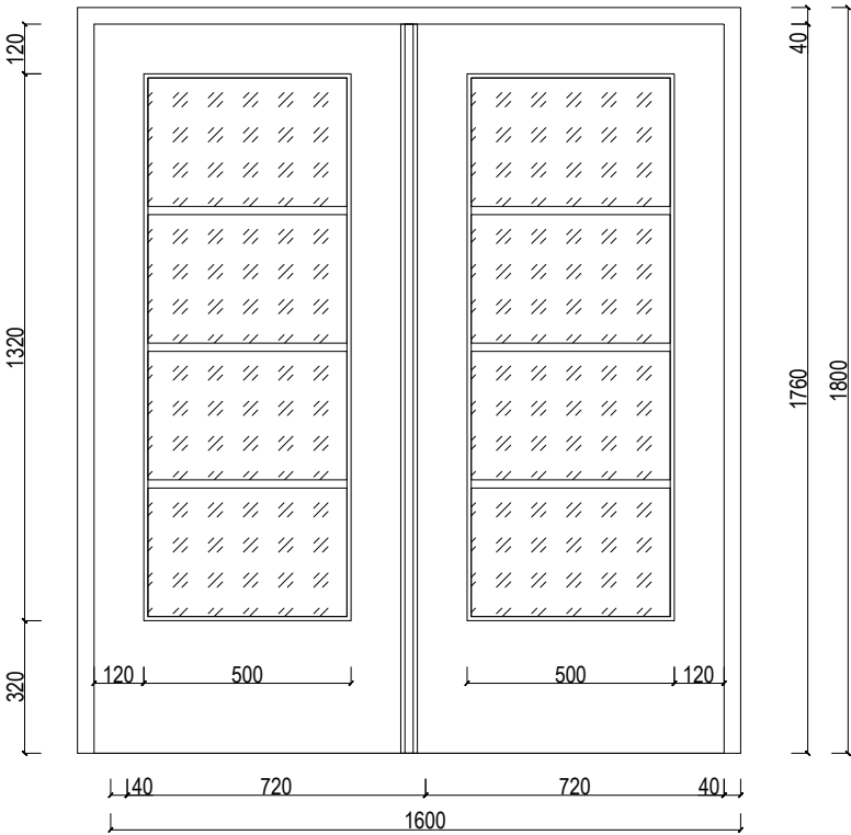
Välisuks VU-4
