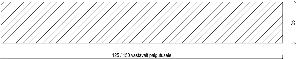
Nurgalauad D-7 M 1:1 toon F461
