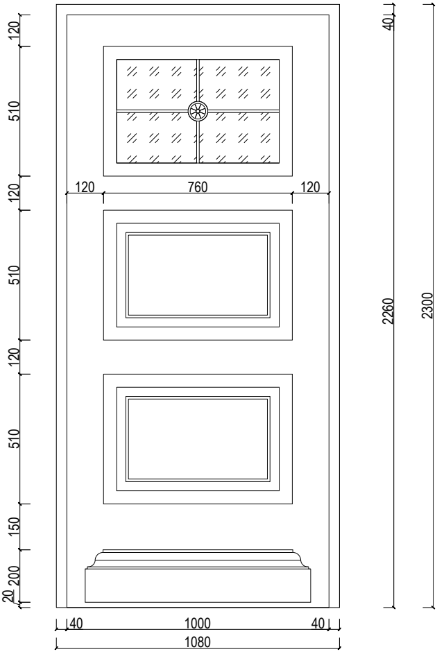
Välisuks VU-1
