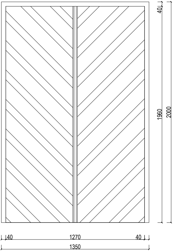
Välisuks VU-5
