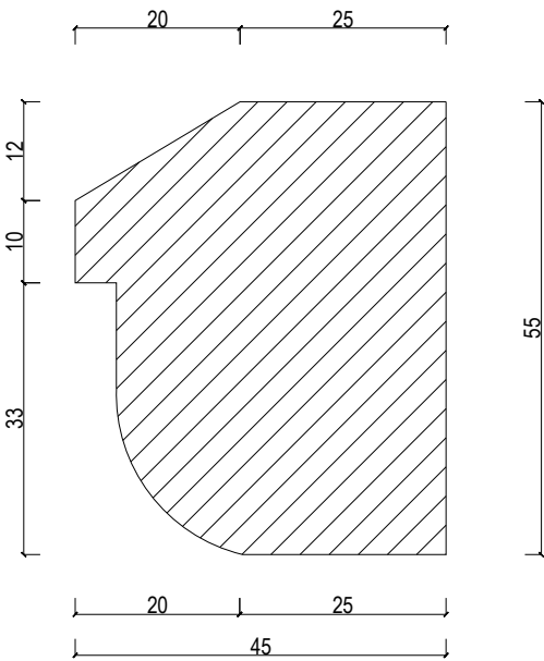
Aknaalune karniis D-9 M 1:1 toon F461
