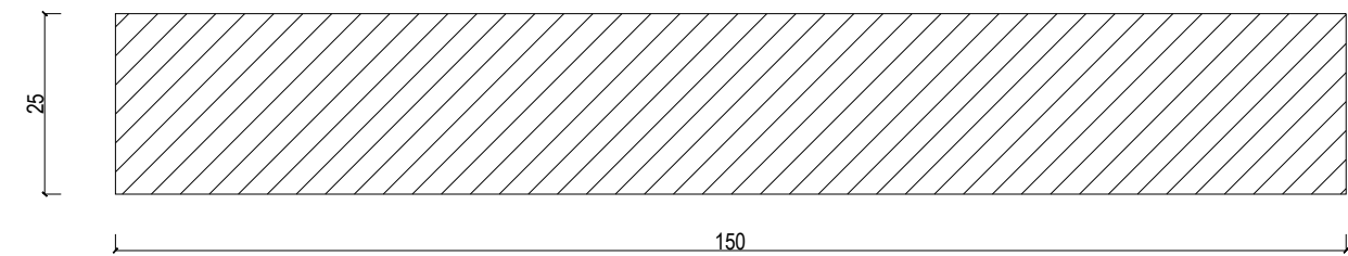
Horisontaalne laudis D-3 (akende vahel) M 1:1 toon J460
