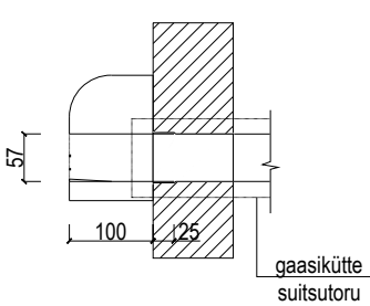
Lõige
