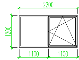
Aken PVC – A2 1tk kolmekordne klaaspakett aknaraamid väljast hall, seest valged
