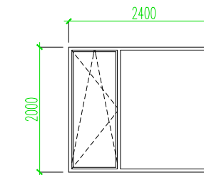
Aken PVC – A14 1tk kolmekordne klaaspakett aknaraamid väljast valge, seest valged
