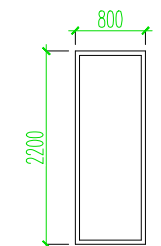
Aken PVC – A10 2tk kolmekordne klaaspakett aknaraamid väljast valge, seest valged
