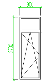
Aken PVC – A15 1tk kolmekordne klaaspakett aknaraamid väljast valge, seest valged
