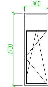
Välisuks – VU2 1tk puidustvälisuks värv valge
