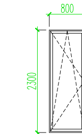
Välisuks – VU4 1tk puidustvälisuks värv valge
