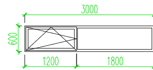
Aken PVC – A3 1tk kolmekordne klaaspakett aknaraamid väljast hall, seest valged
