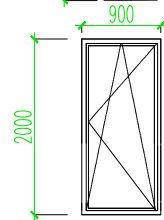
Aken PVC – A5 3tk kolmekordne klaaspakett aknaraamid väljast valge, seest valged
