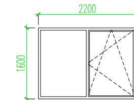
Aken PVC – A7 2tk kolmekordne klaaspakett aknaraamid väljast valge, seest valged
