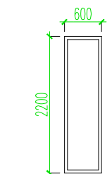
Aken PVC – A9 1tk kolmekordne klaaspakett aknaraamid väljast valge, seest valged
