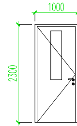
Välisuks – VU1 1tk puidustvälisuks värv valge
