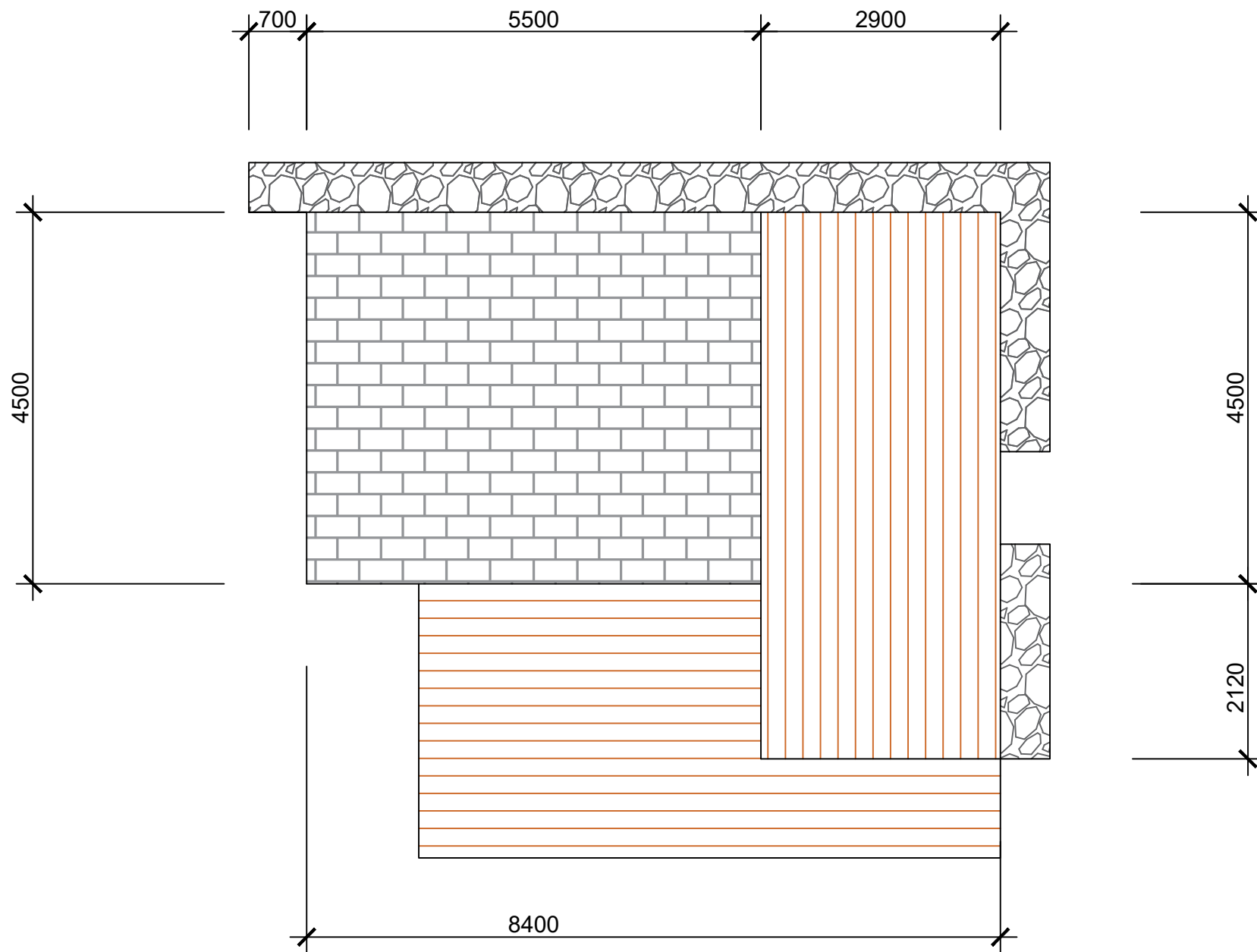
Põranda plaan
