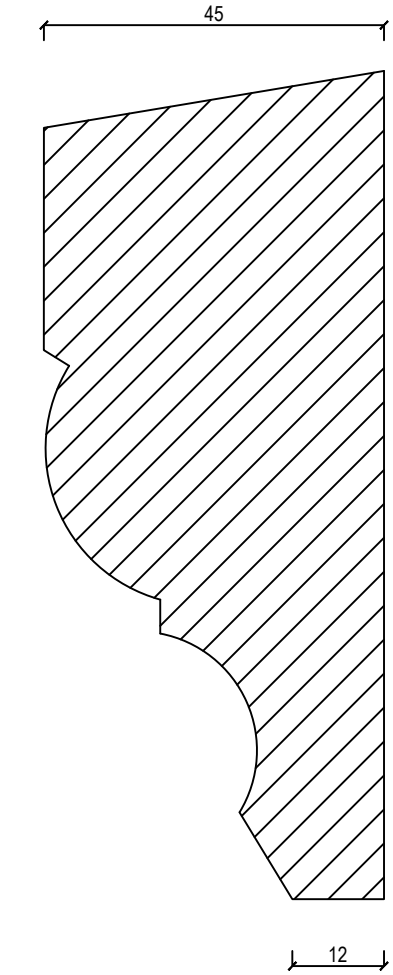
Aknapealne ja -alune karniis D-6 M 1:1
