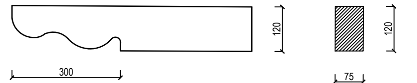
Saelõikelised sarikaotsad D-12 (projekteeritud detail katusepealsetele vintskappidale) M 1:10
