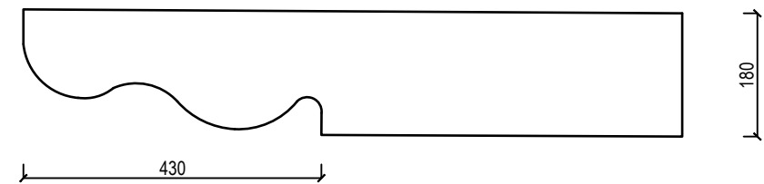
Saelõikelised sarikaotsad D-12 (projekteeritud detail katusepealsetele vintskappidale) M 1:10
