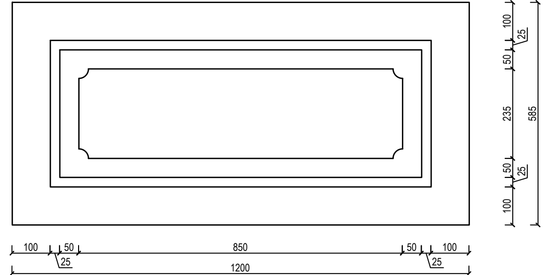
Dekoratiivne plaat II korruse akende all D-10 (olemasolev originaaldetail) M 1:2
