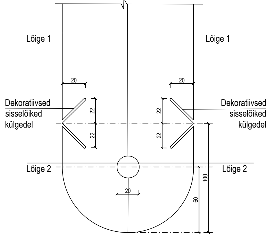
Vertikaalne otsalaud D-8 (olemasolev originaaldetail) M 1:2
