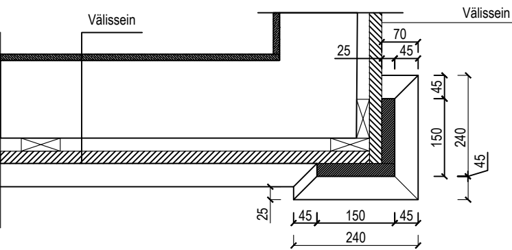
Karniiside pööre hoone otsaseinale (hoone nurgas) M 1:10
