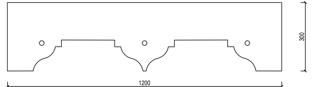
Saelõikelised sarikaotsad D-11 (olemasolev originaaldetail) M 1:10
