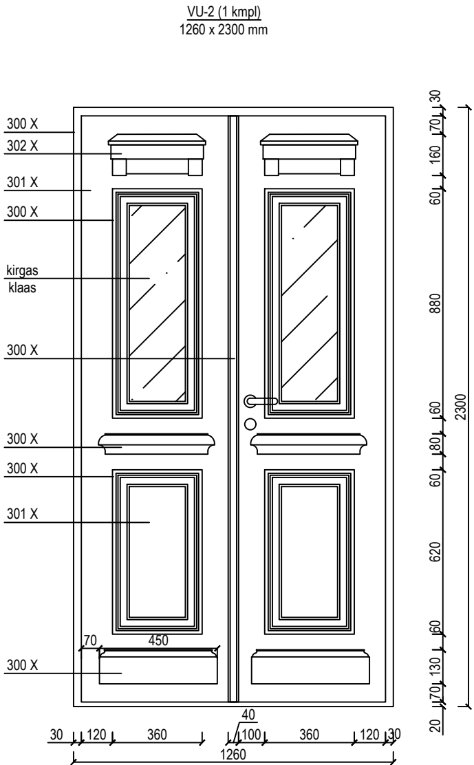
VU-2 - olemasolev välisuks. Korrastada, värvida etteantud toonides.
