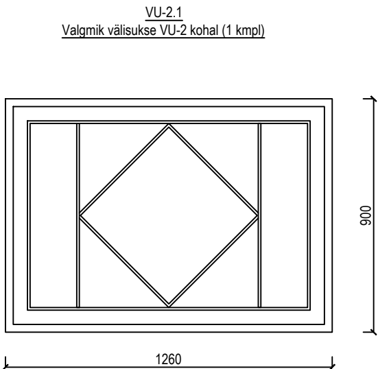
VU-2.1 - olemasoleva ukse kohal paiknev valgmik. Korrastada, värvida etteantud toonides. Puitraam, kirgas klaas.
