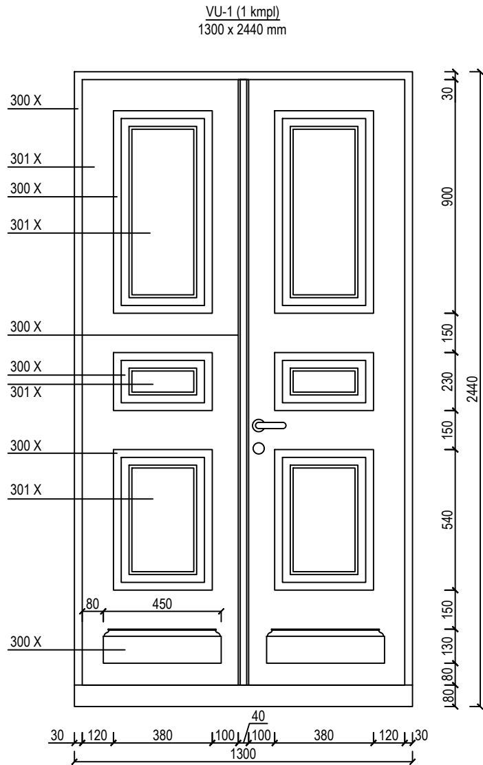
VU-1 - olemasolev välisuks. Korrastada, värvida etteantud toonides.
