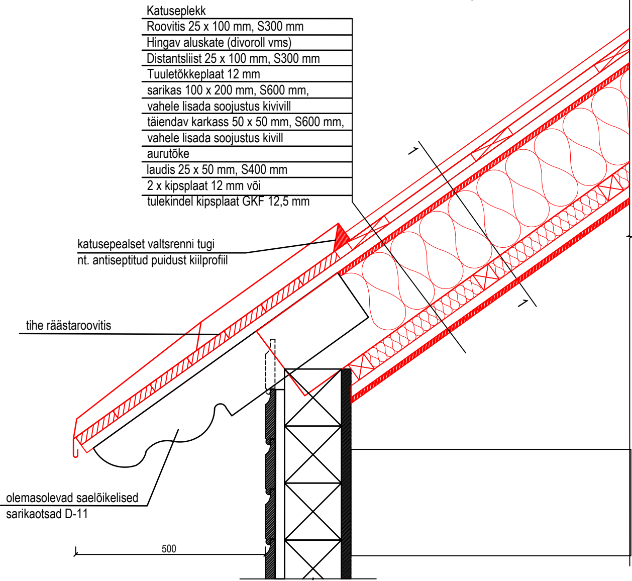
Katuse lõige 1-1 M 1:10
