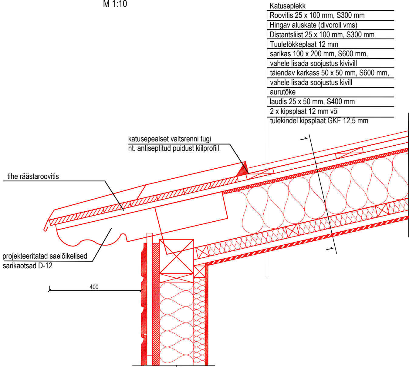
Katuseräästa sõlm. Katusepealsed vintskapid M 1:10
