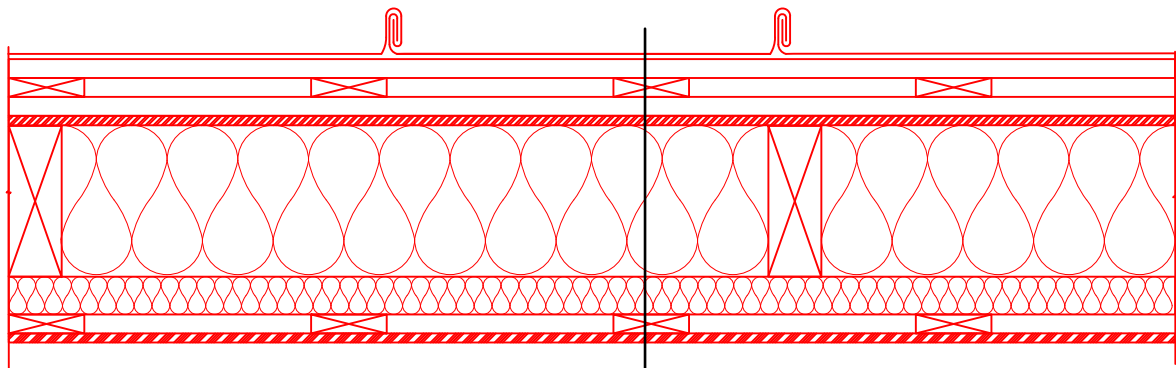
Katuse lõige 1-1 M 1:10
