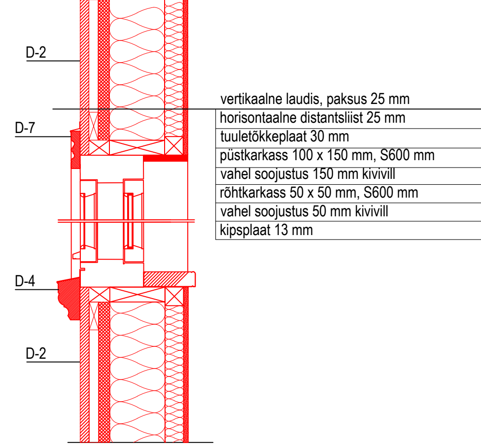
Akende paiknemine projekteeritava vintskapi välisseinas Vertikaallõige M 1:10
