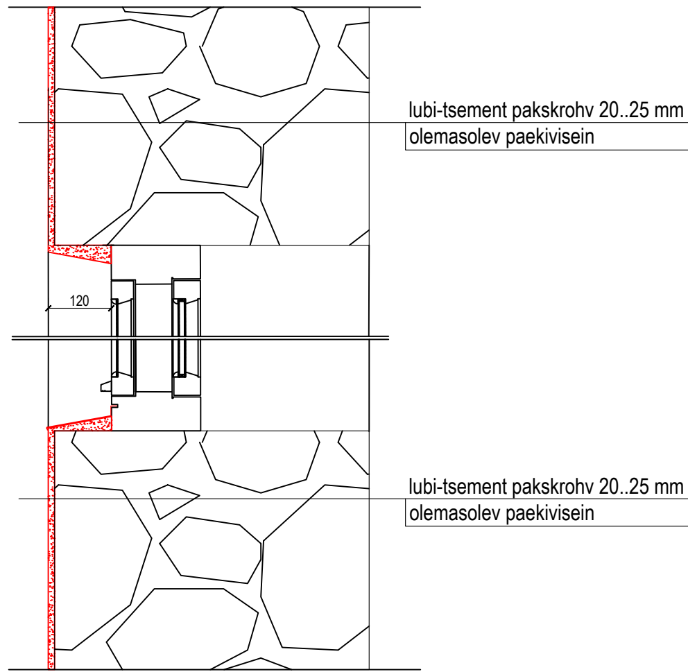
Akende paiknemine krohvitas sokli seinas. Horisontaallõige M 1:10
