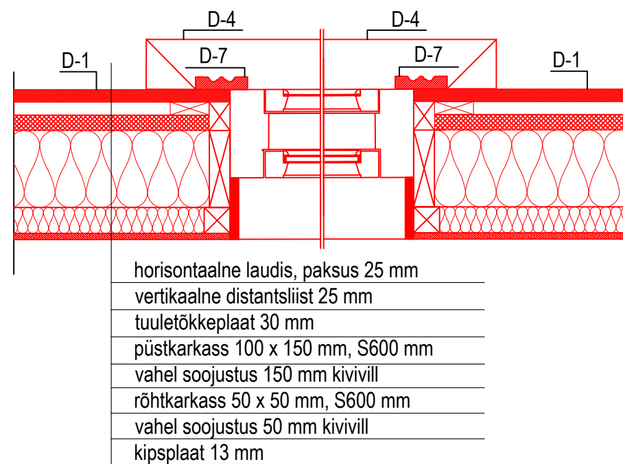
Akende paiknemine projekteeritava vintskapi välisseinas Horisontaallõige M 1:10
