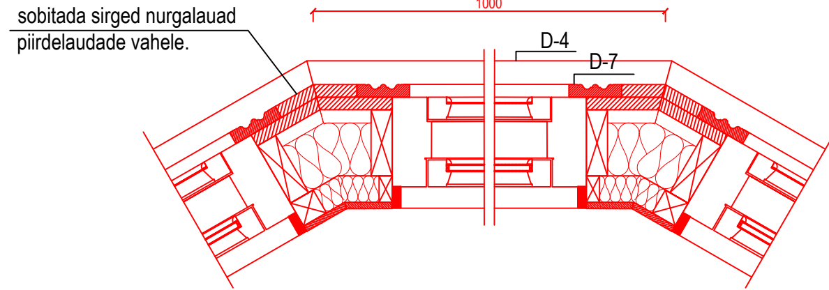
Akende paiknemine taastatava torni välisseinas Horisontaallõige M 1:10
