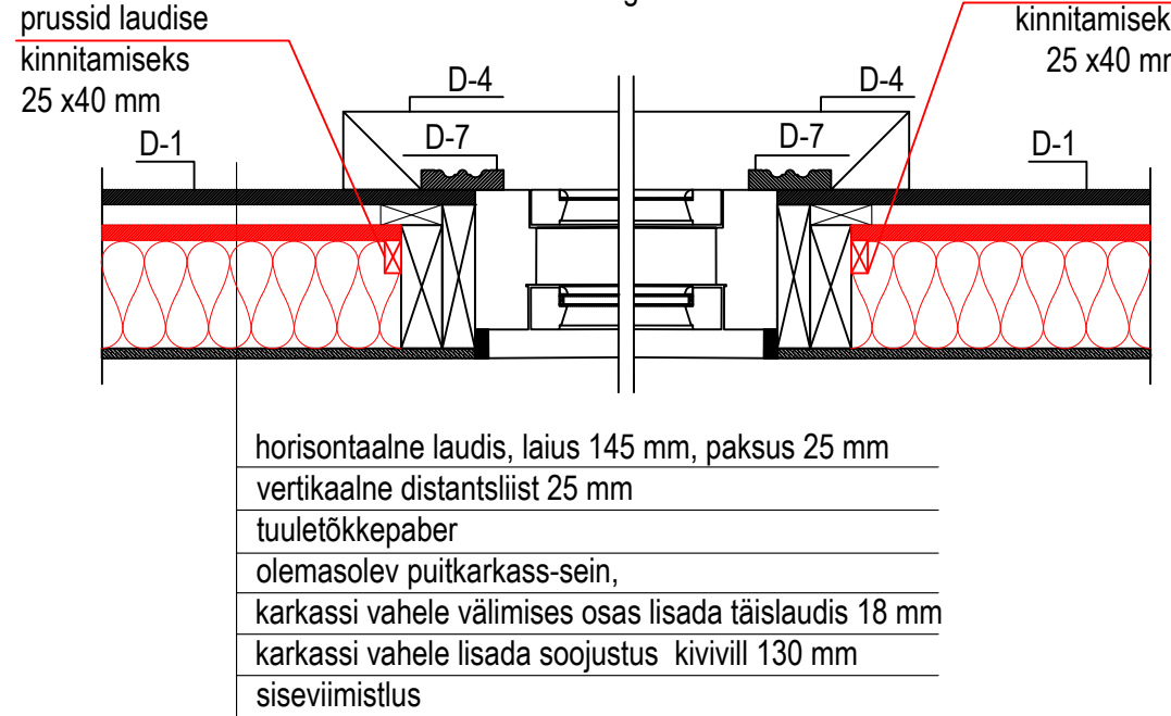
Akende paiknemine otsaseinas (hoovipoolne trepikoda). Horisontaallõige M 1:10
