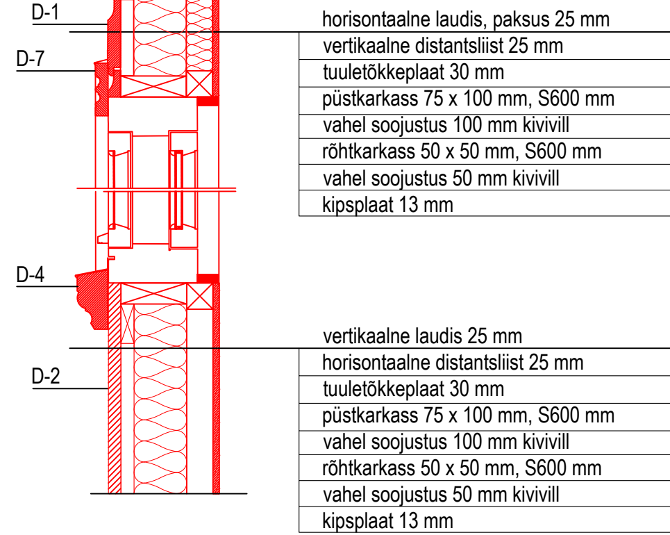
Akende paiknemine taastatava torni välisseinas Vertikaallõige M 1:10
