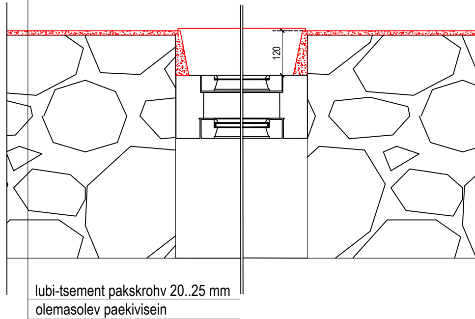
Akende paiknemine krohvitas sokli seinas. Horisontaallõige M 1:10
