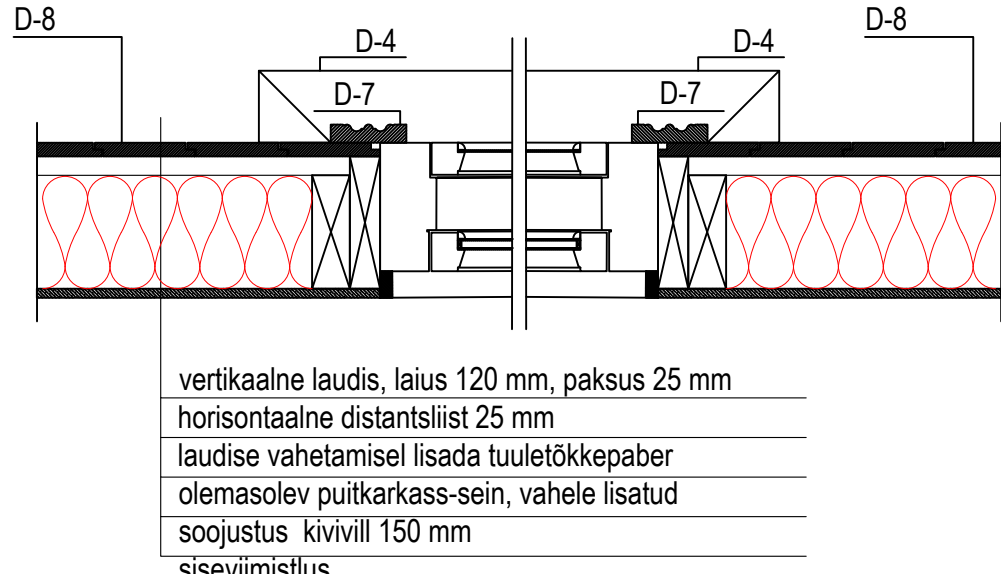
Akende paiknemine otsaseinas (v.a. hoovipoolne trepikoda). Horisontaallõige M 1:10
