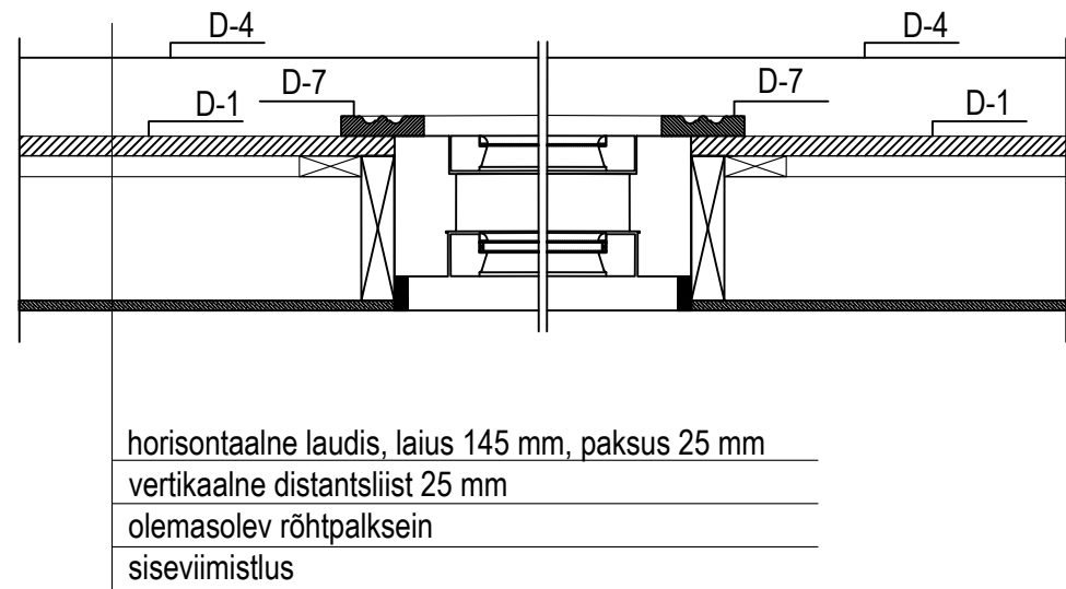
Akende paiknemine välisseinas. Horisontaallõige M 1:10
