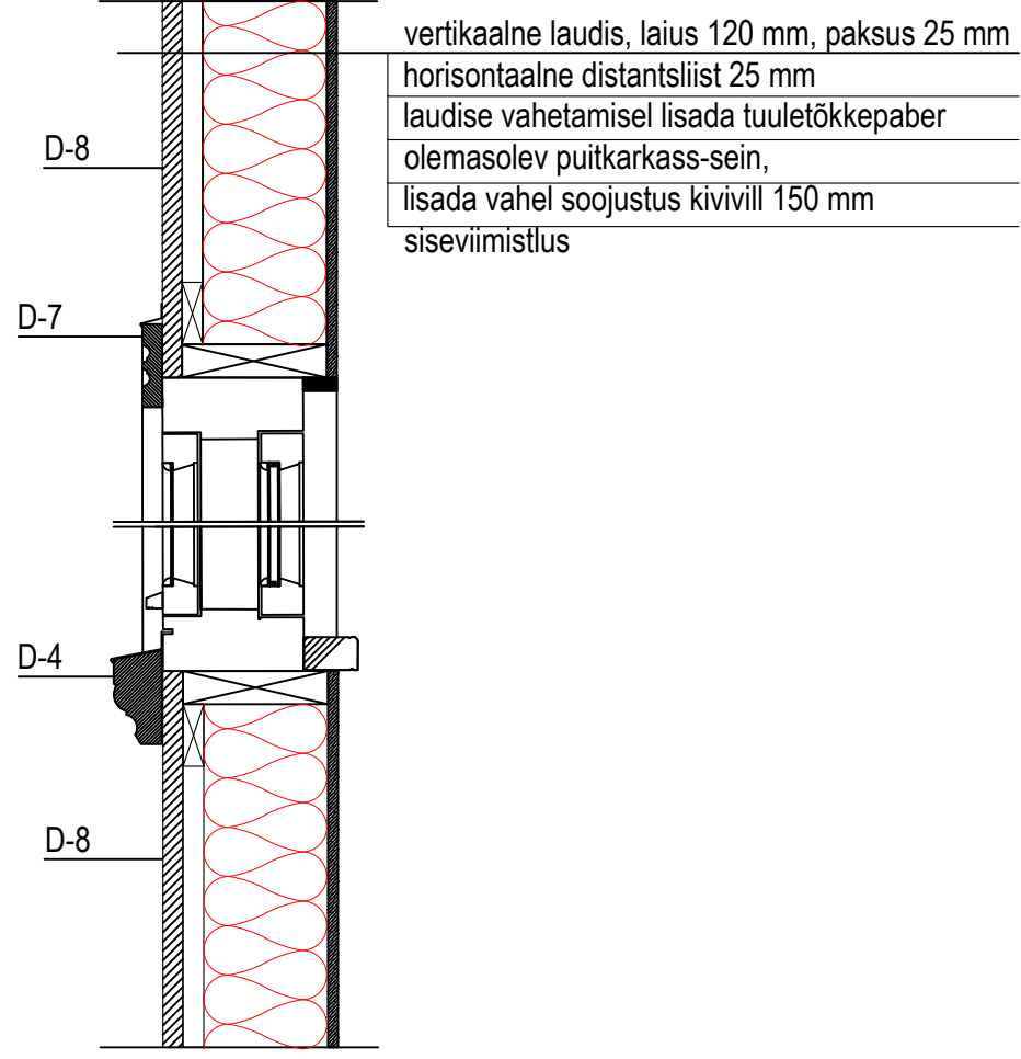
Akende paiknemine otsaseinas (v.a. hoovipoolne trepikoda). Horisontaallõige M 1:10
