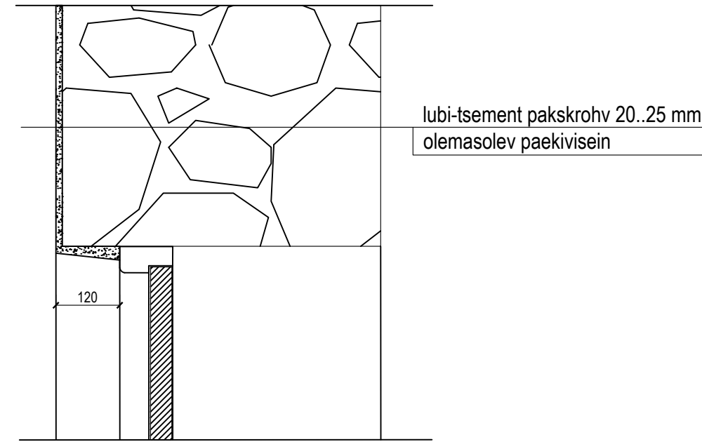
Välisukse VU-5 paiknemine sokli seinas. Vertikaallõige M 1:10
