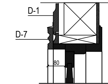
Välisuste paiknemine puitseinas seinas. Horisontaallõige M 1:10
