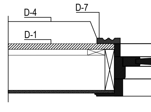
Välisuste paiknemine puitseinas seinas. Horisontaallõige M 1:10
