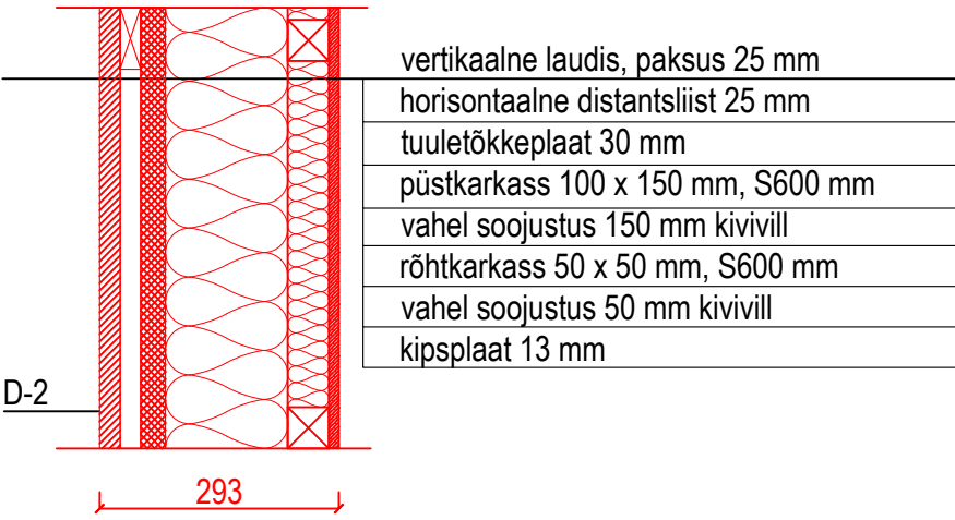
Projekteeritava katusepealse vintskapi sein M 1:10
