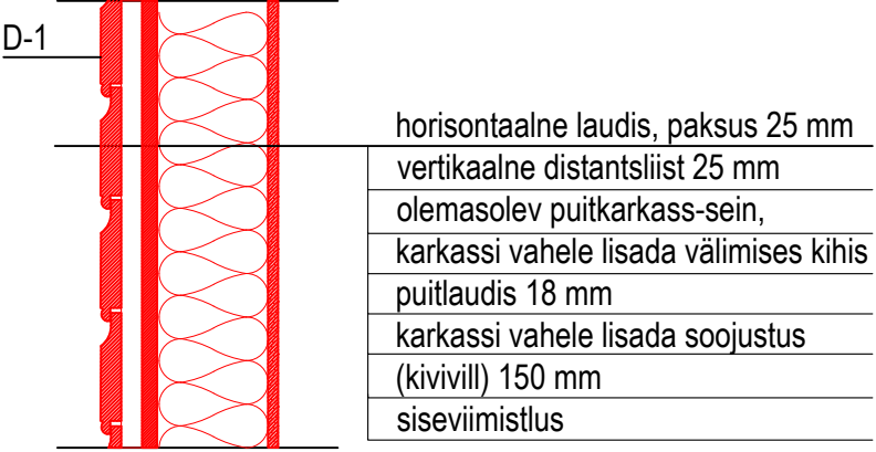
Viilualune otsasein (hoovipoolne trepikoda) M 1:10
