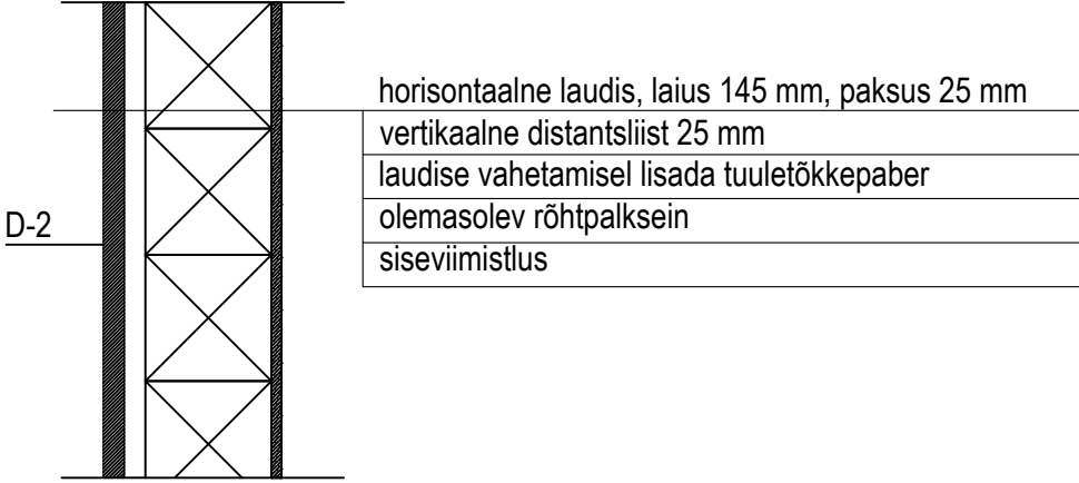
Välissein (vertikaalne laudis) M 1:10
