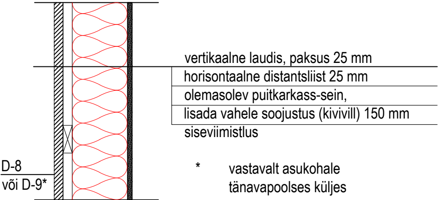
Viilualune otsasein (v.a. hoovipoolne trepikoda) M 1:10
