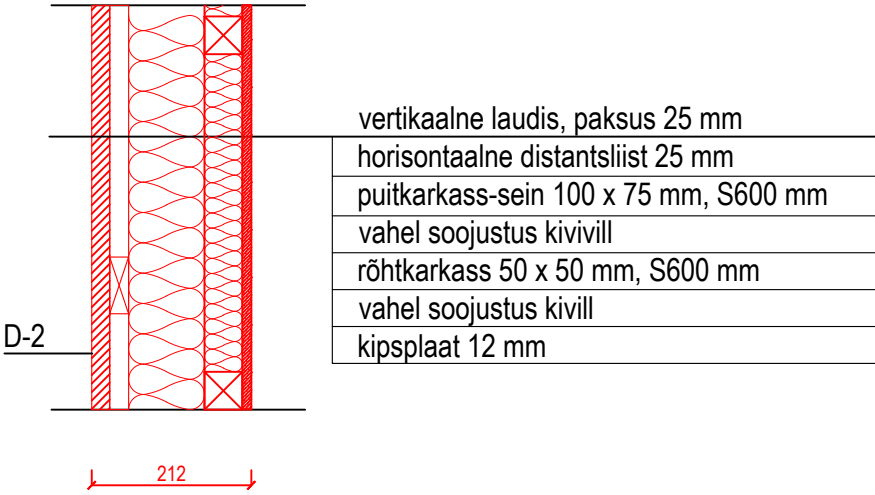
Projekteeritava katusepealse vintskapi sein M 1:10
