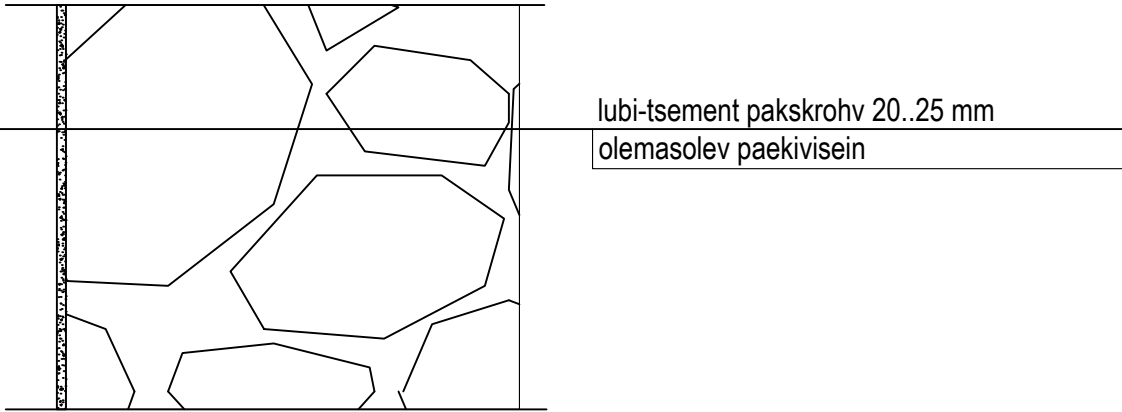
Sokli sein M 1:10
