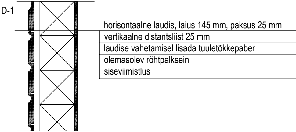
Välissein (horisontaalne laudis) M 1:10
