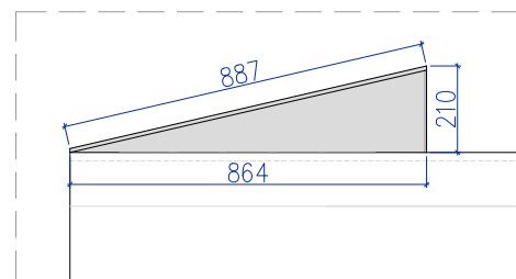
TREPIKOJA KATUSE PÕHIMÖTTELINE KUJU VAADE B
