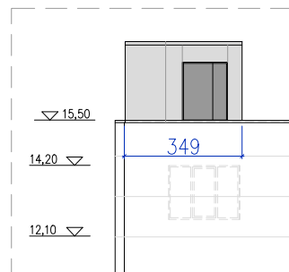
TREPIKOJA KATUSE PÕHIMÖTTELINE KUJU VAADE A
