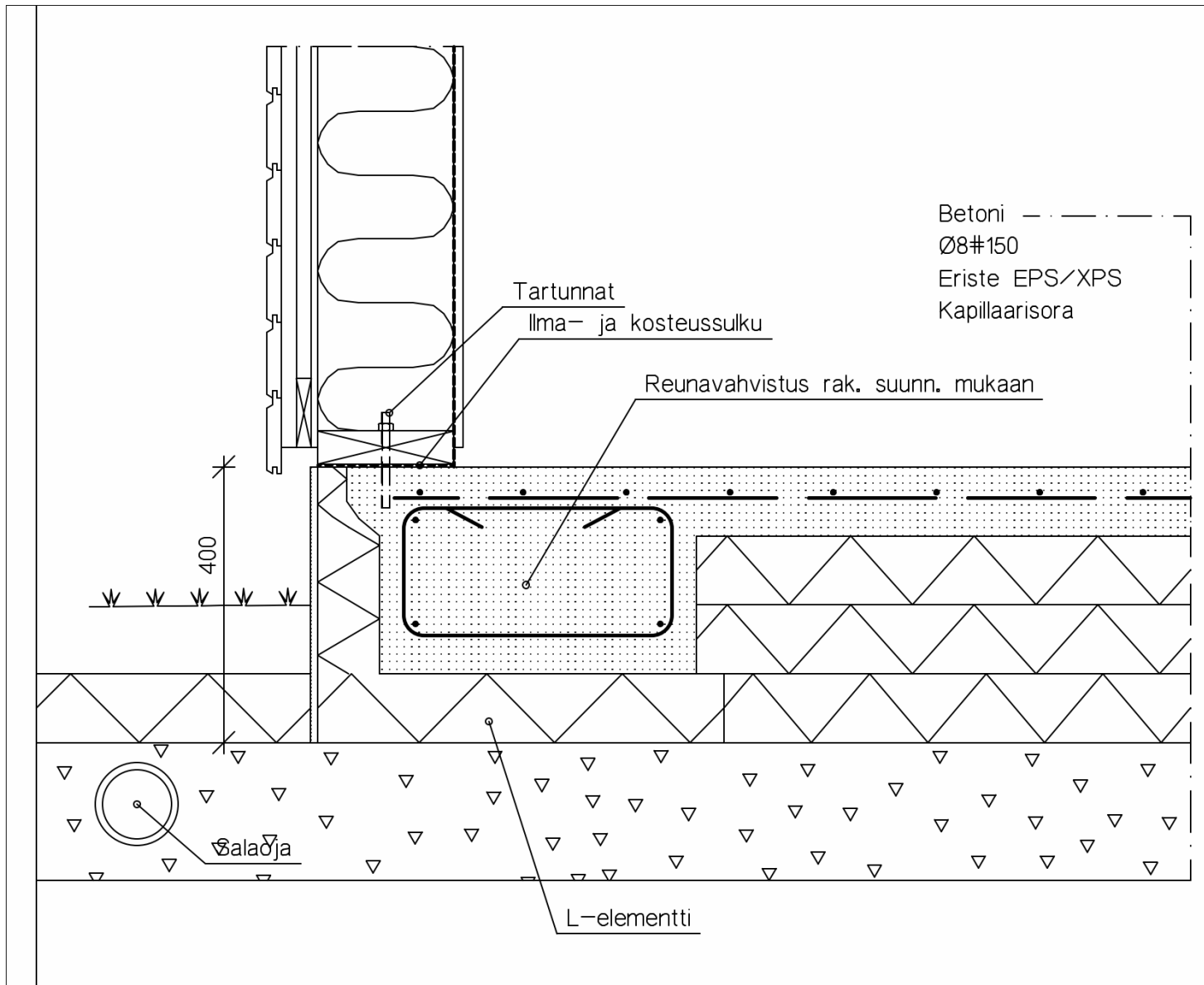
L-Sokkelielementti 400 mm
