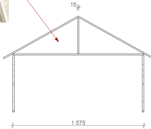
NELIKANT-TERASLATIST VARJUALUNE
