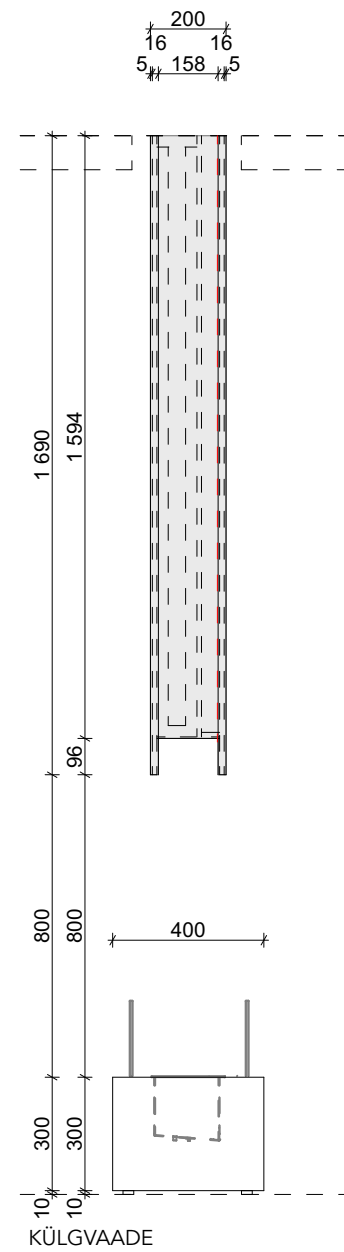
KÜLGVAADE
