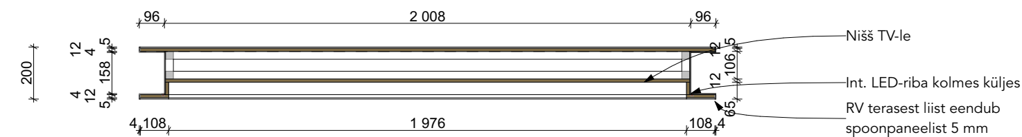
LÕIGE A-A
