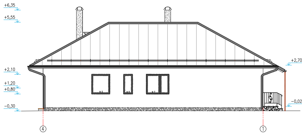
VAADE LÕUNAST
