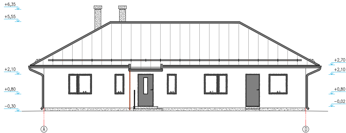
VAADE IDAST
