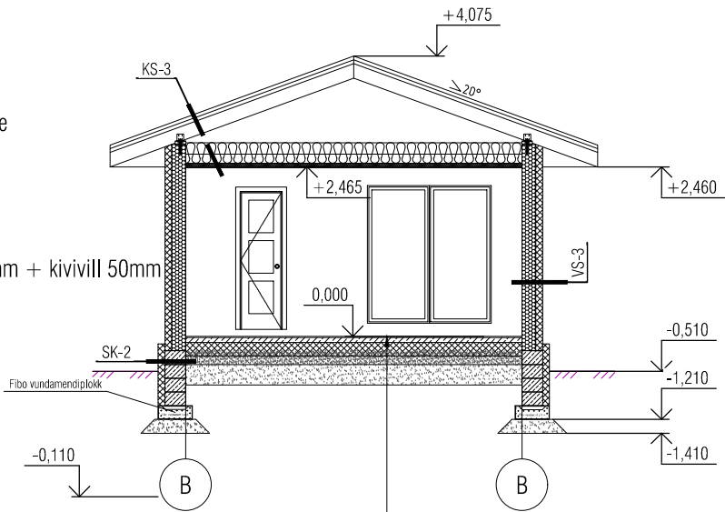
LÕIGE 1-1
