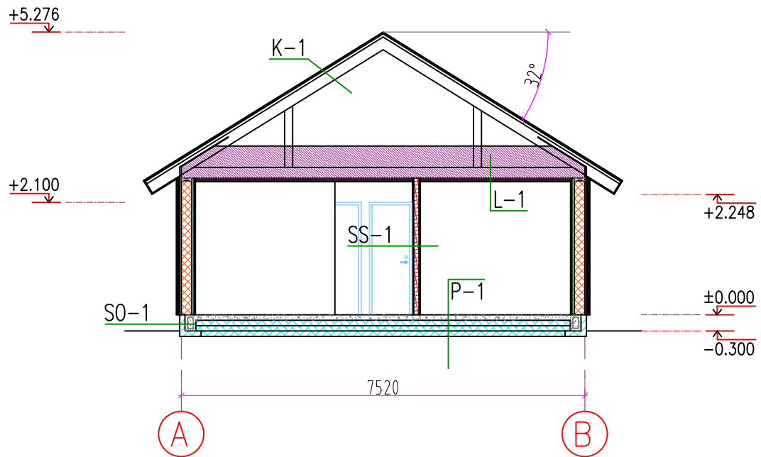
Lõige A-A
