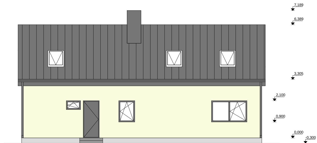
Vaade C
