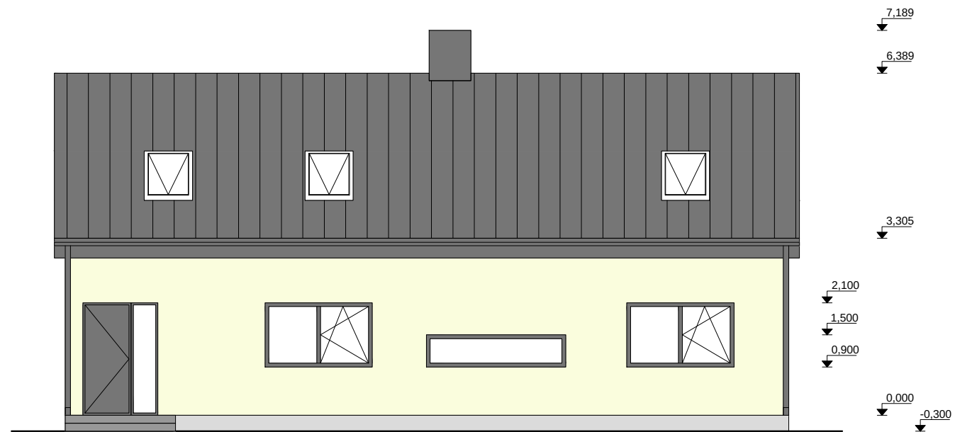
Vaade A
