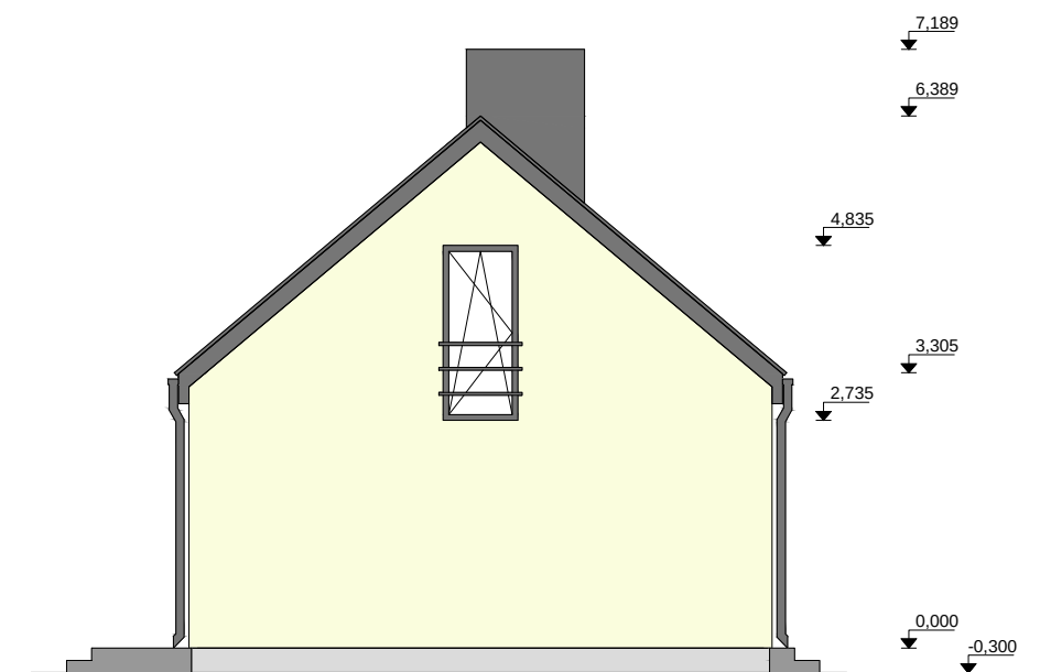
Vaade D
