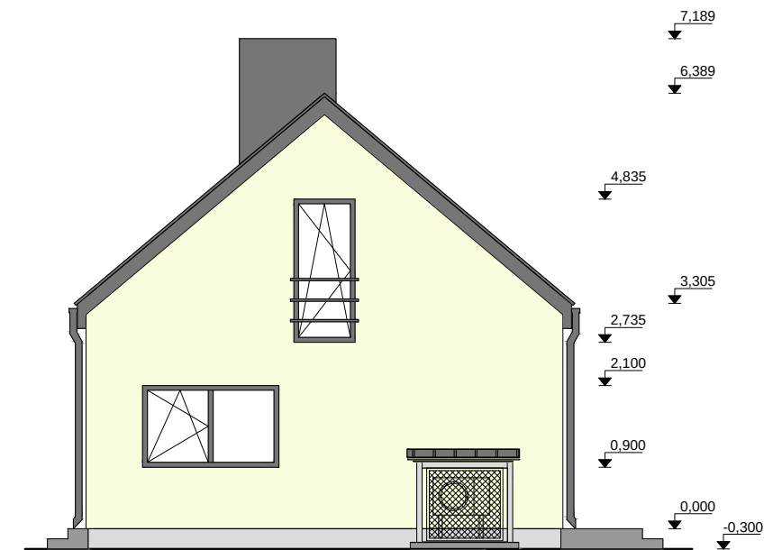
Vaade B
