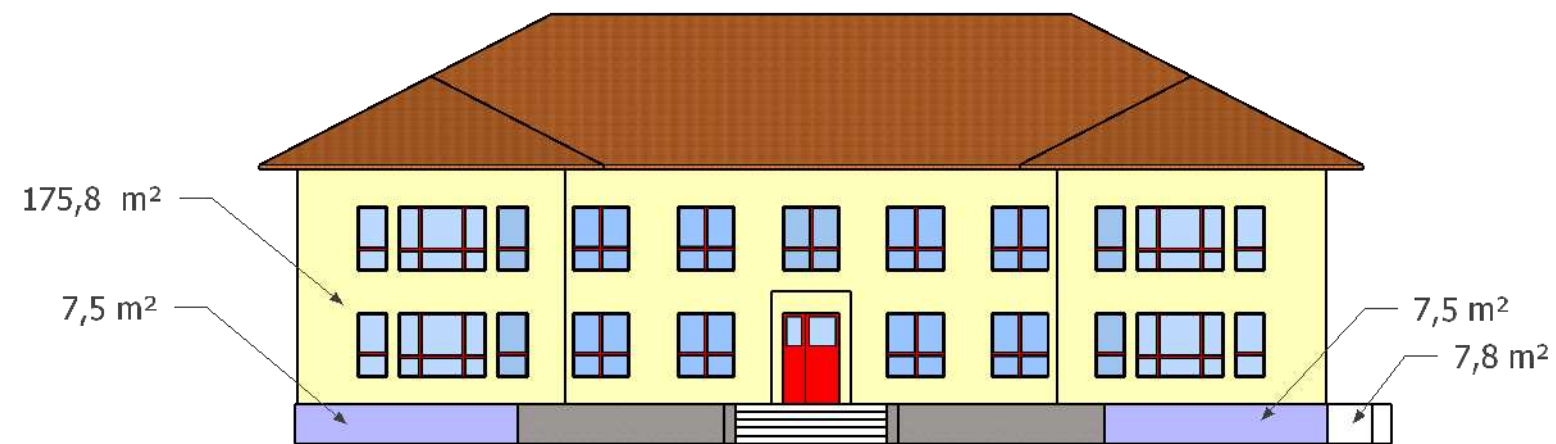
Esifassaad
