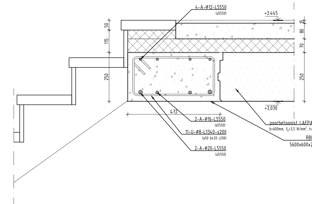
VLS-09 M1:10
