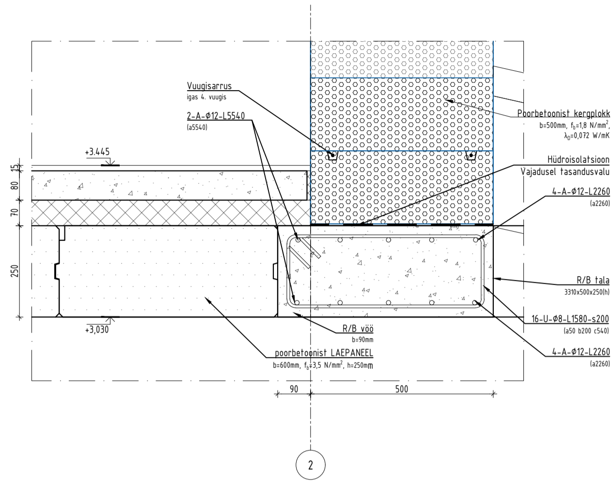
VLS-01 M1:10
