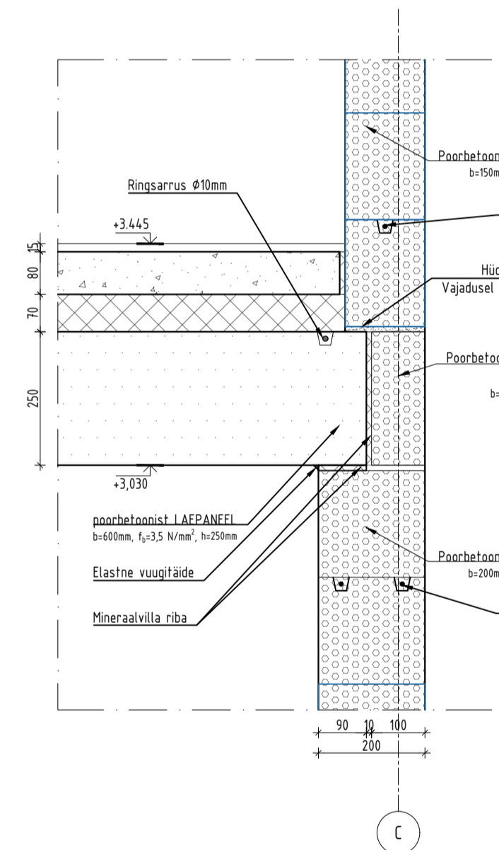
VLS-06 M1:10
