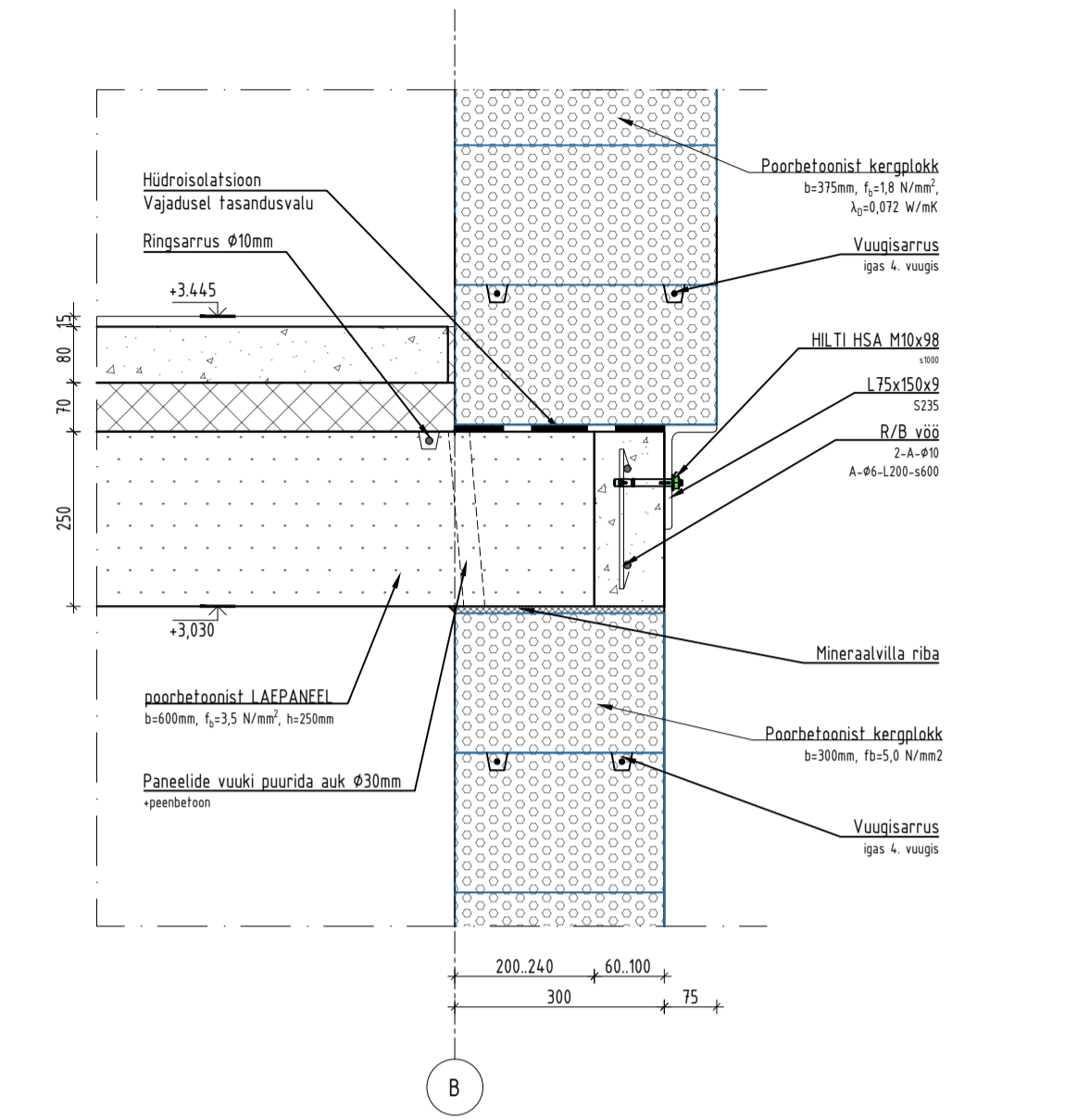
VLS-04 M1:10
