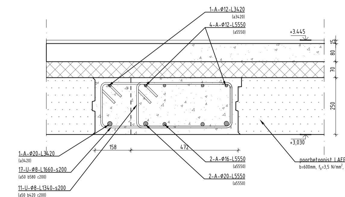
VLS-09 M1:10
