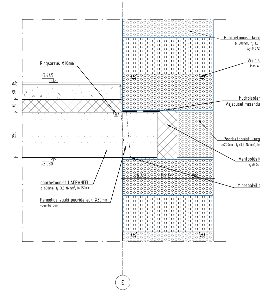
VLS-03 M1:10
