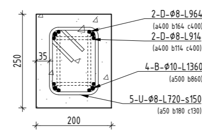
VUS 06. Lõige 4-4 M1:10
