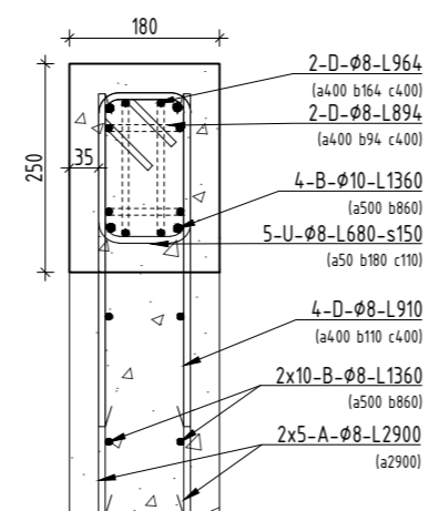
VUS 06. Lõige 2-2 M1:10
