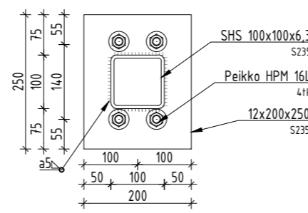
VUS 06. Lõige 4-4 M1:10
