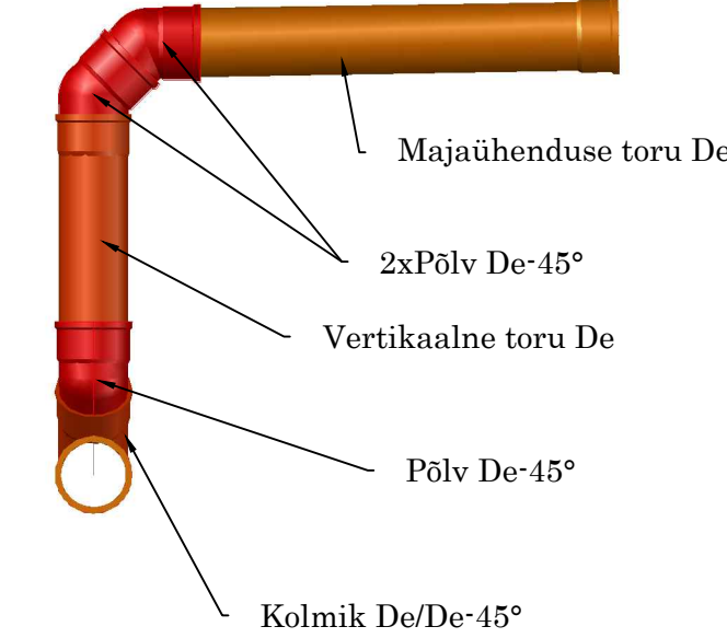
Pimeühendus tüüp 1 vertikaalse toruga
