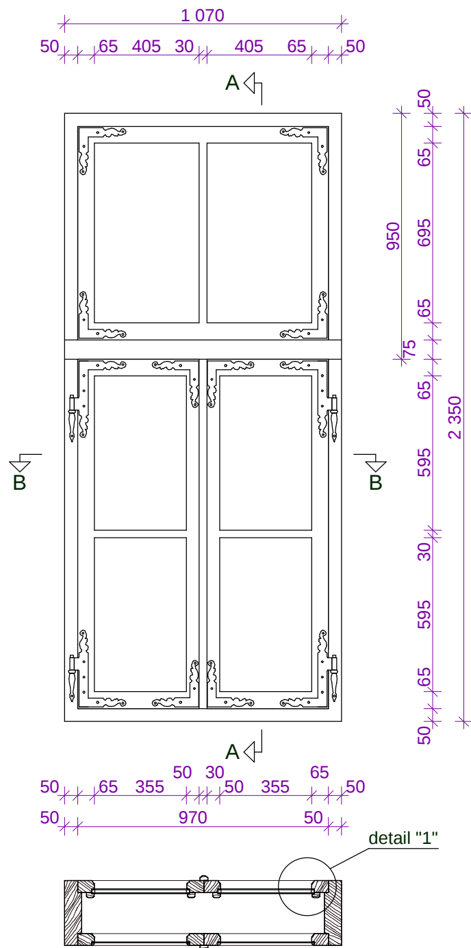
Lõige B - B
