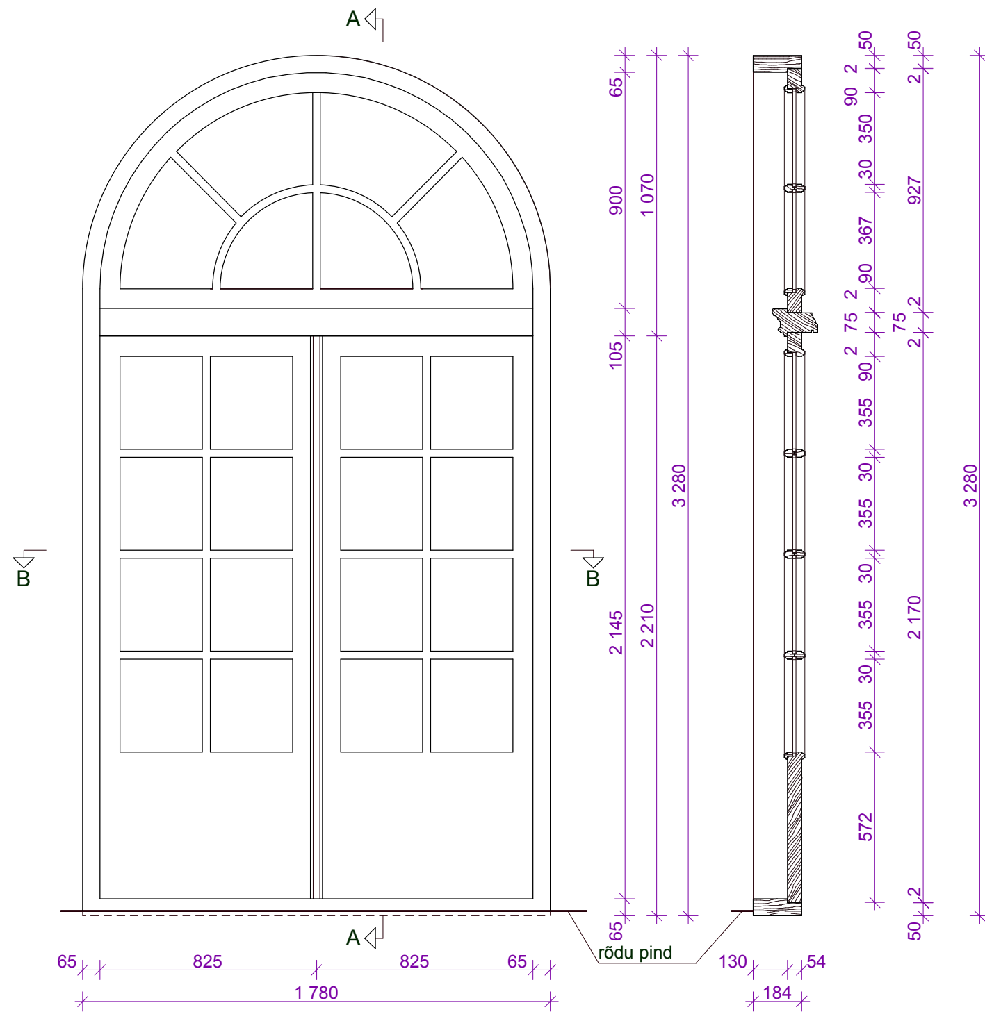
Lõige A - A
