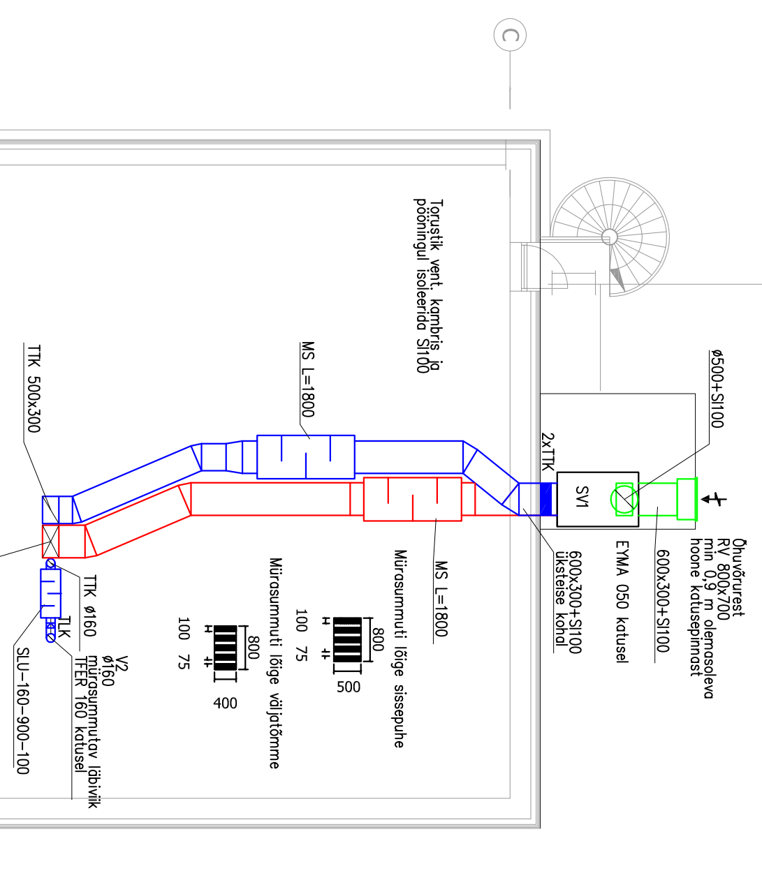
Pöningukorruse põhim. ventilatsiooniplaan ja lõige
