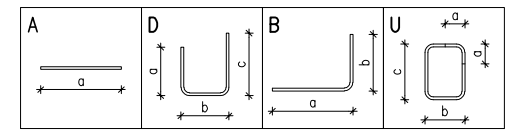
Sarruse painutustüübid
