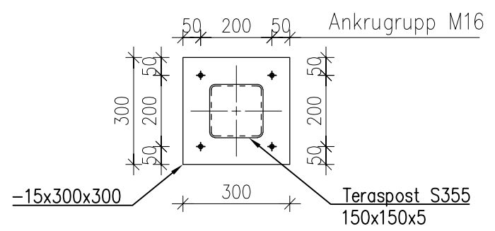
1-1 (ankrurupp M16) M1:15
