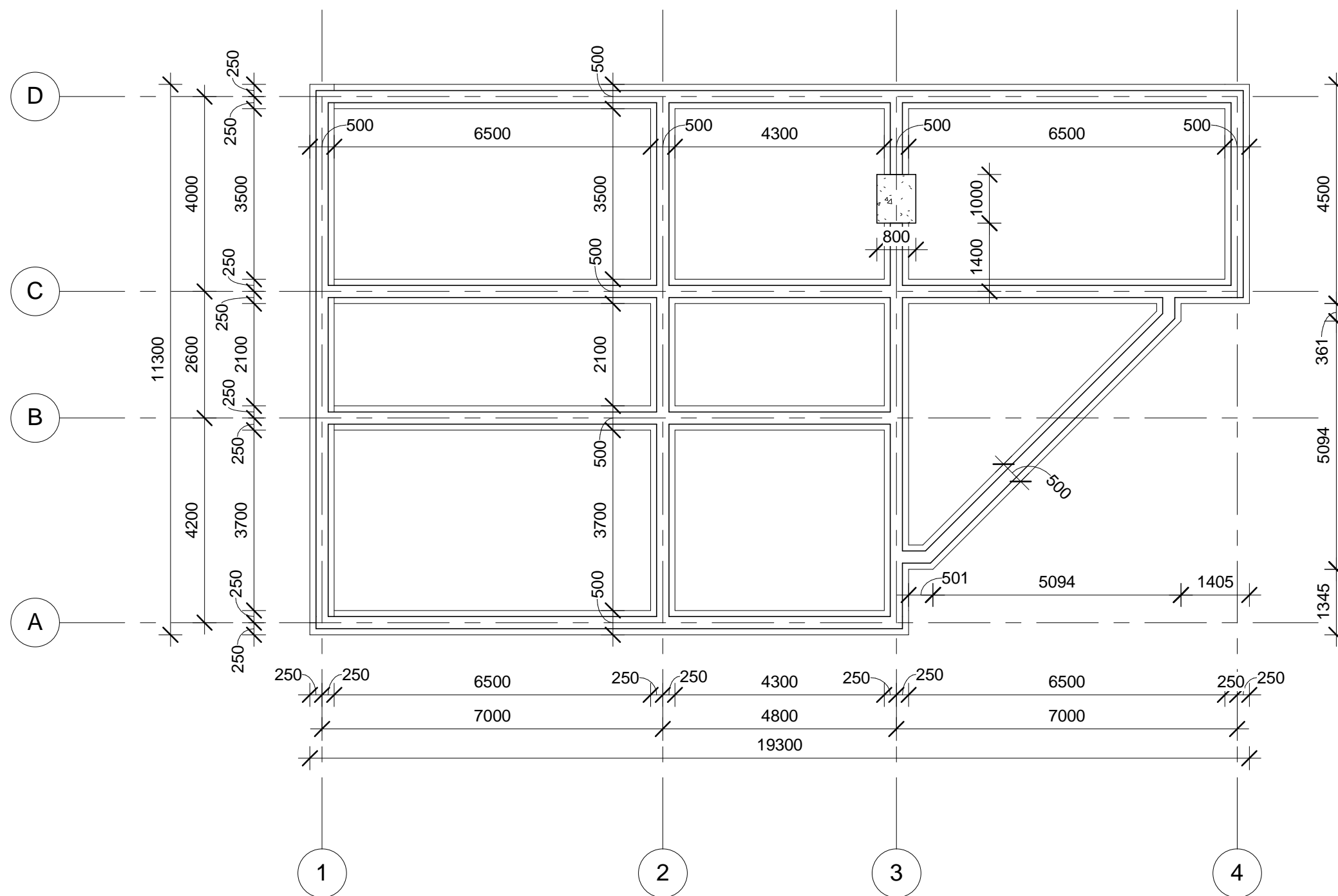
1 Vundamendi plaan 1 : 100
