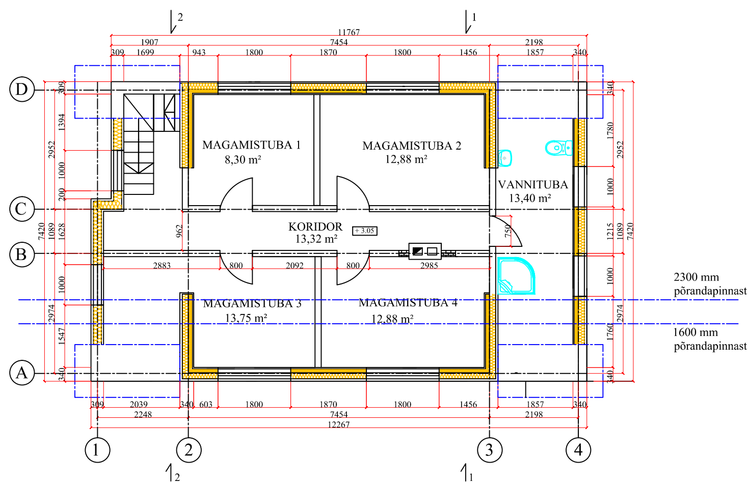
KATUSEKORRUSE PLAAN
