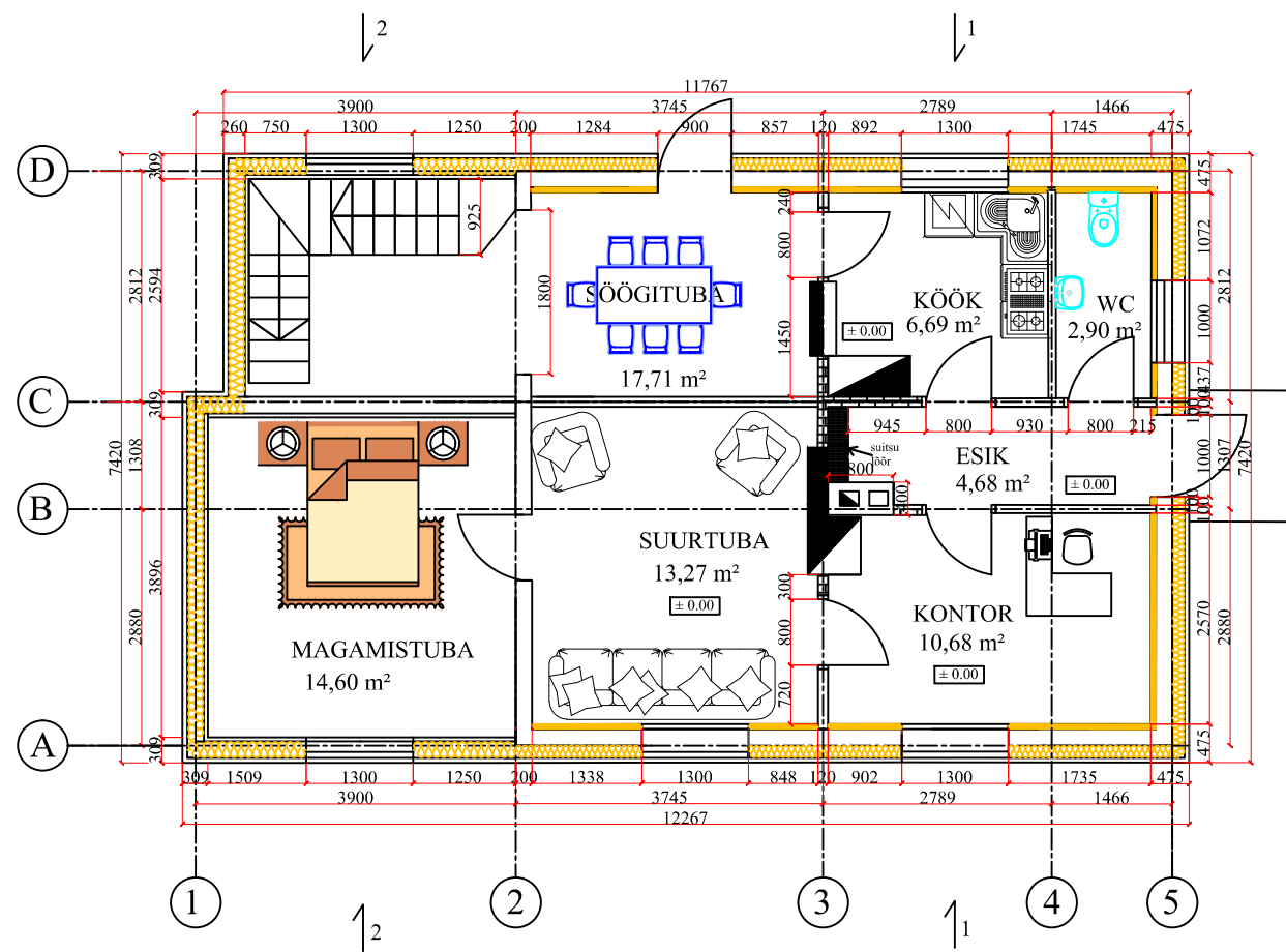
PÕHIPLAAN
