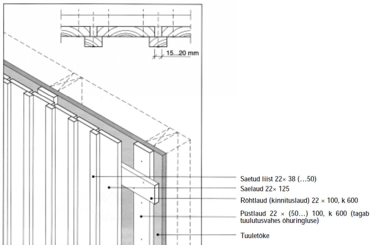
Joonis 9. Katteliistudega laudise näide, rõhtlõige 1:5 ja aksoneetria
