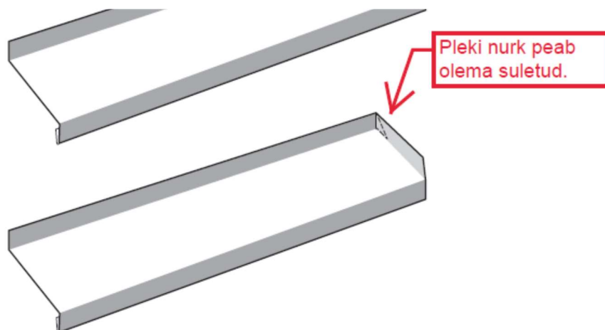
Joonis 27. Avakülje kaitseplekk, selle liitumine aknaplekiga ja ülaliist
