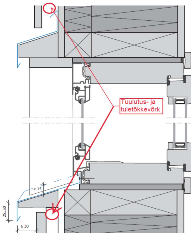
Joonis 19. Aknapleki kinnitamine puitakna piida külge. Plekiserva ülespööre piidale või muule külgnevale pinnale on vähemalt 15 mm
