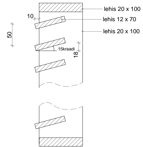
SÕLMED M1:5
