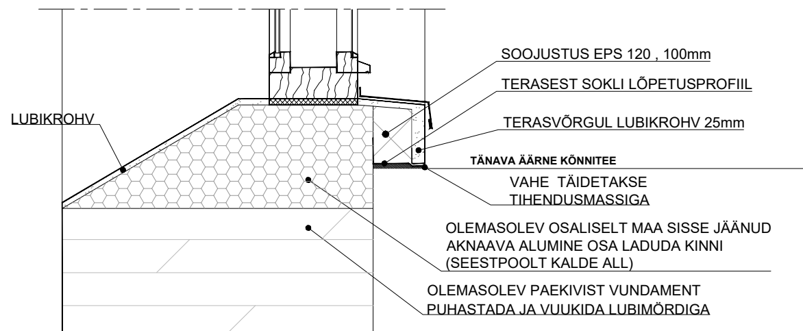
SÕLM 4-4 M1:10
