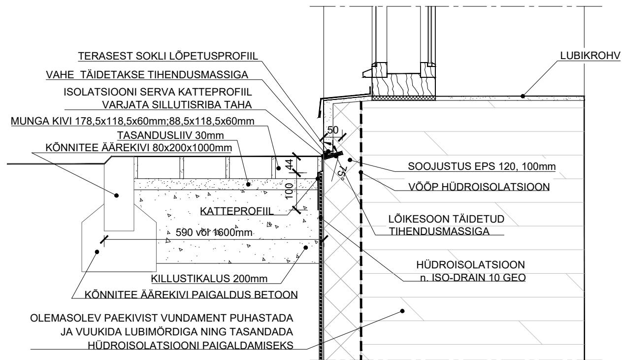
SÕLM 3-3 M1:10
