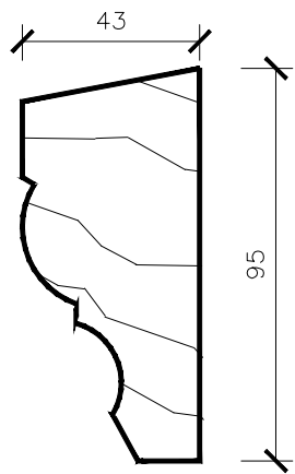
PUIDUST KARNIISILIIST LKAR 43X95mm
