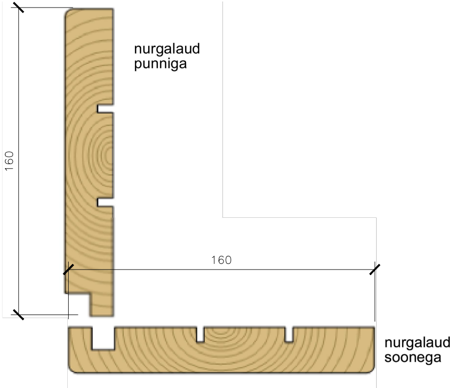
PÕHIMAHU NURGALAUAD 18x160mm
