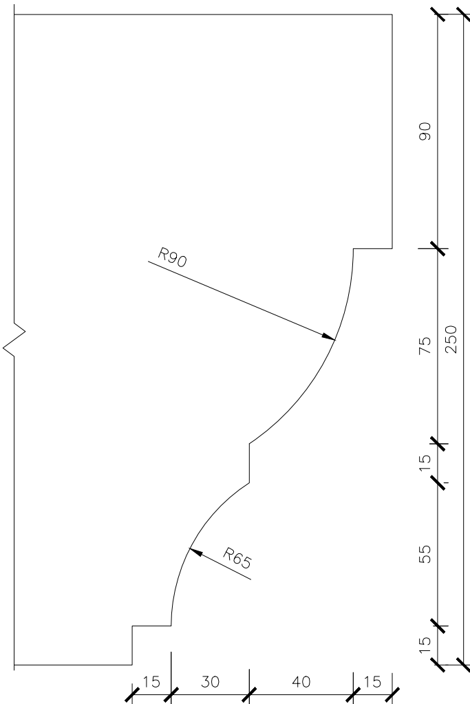
PÄRLINIOTS 150x250mm
