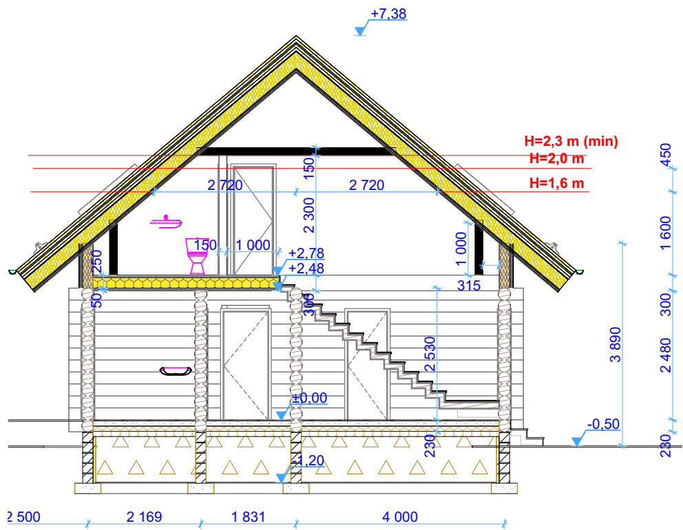
Lõige 1
