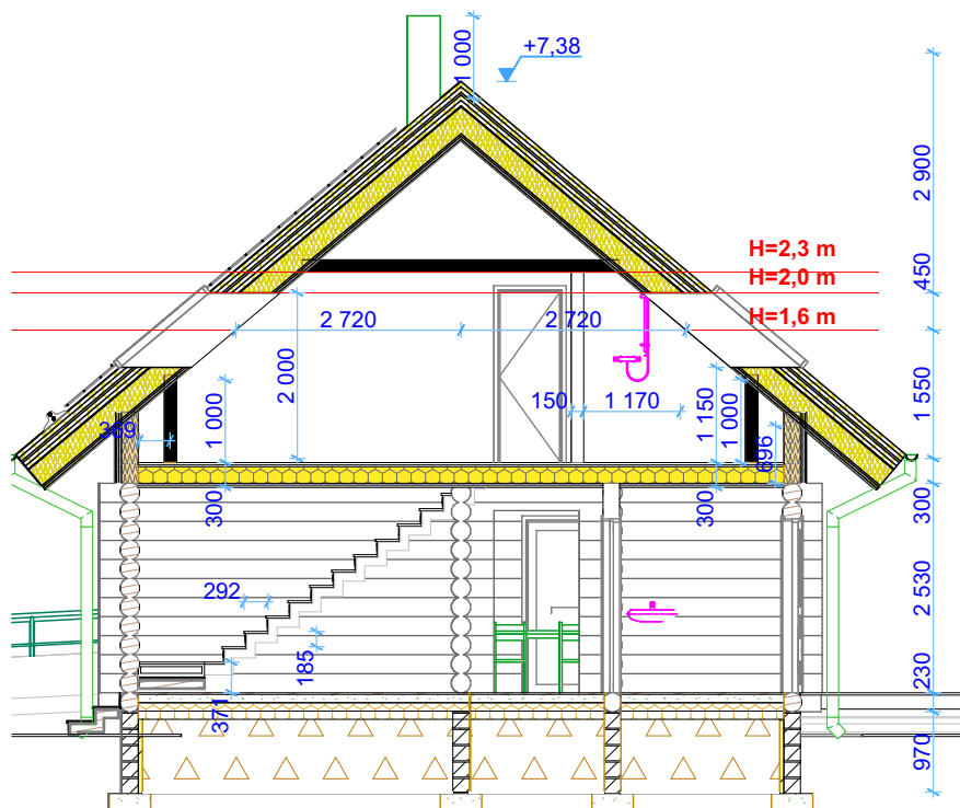
Lõige 1
