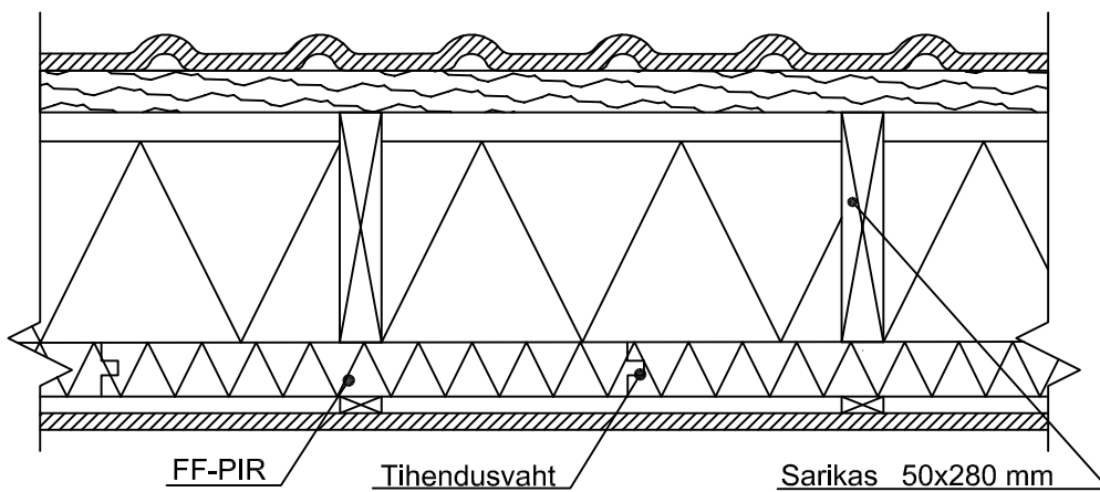
HORISONTAALLÕIGE 1-1
