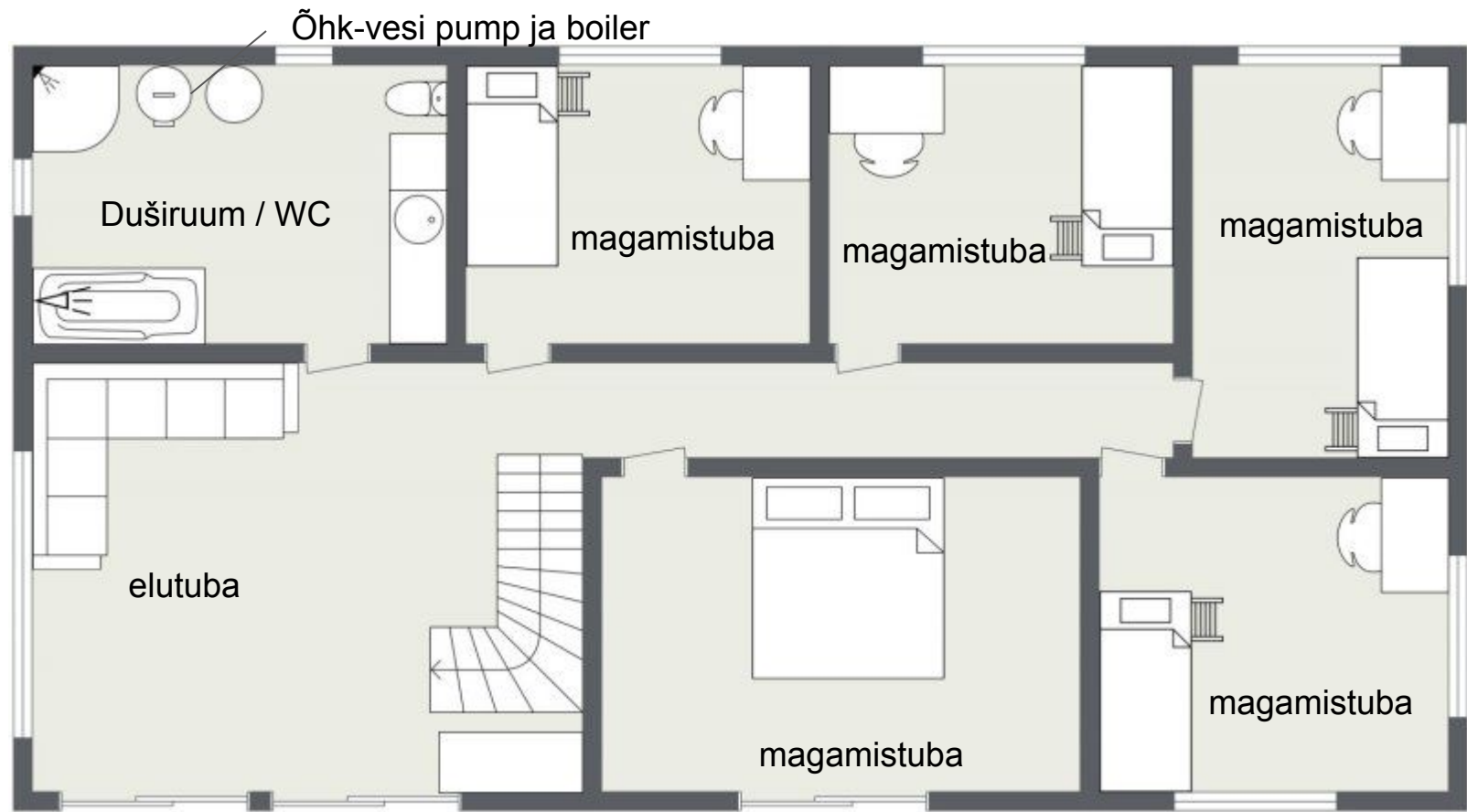
2. korrus
