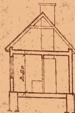
LÕIGE-A-A
