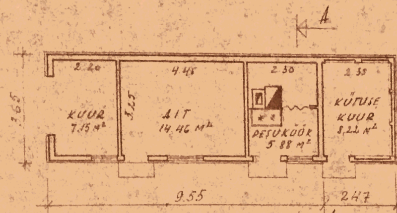
PÕRIPLAAN
