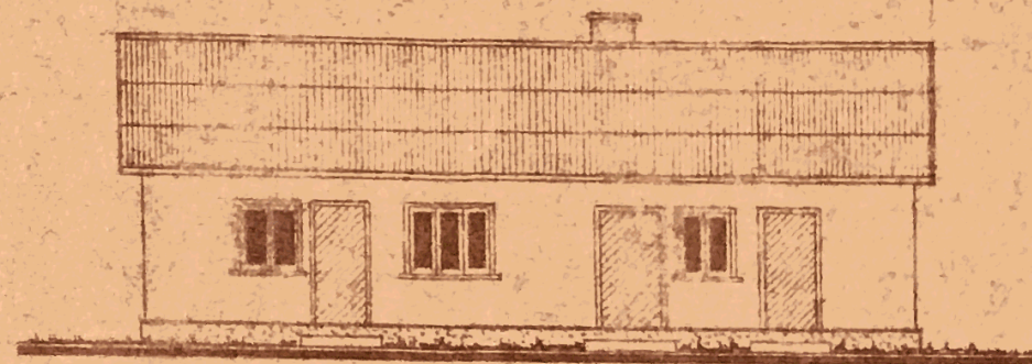
EESTIVAADE
