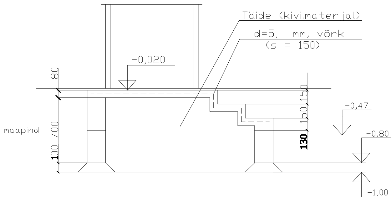
Lõige 1-1
