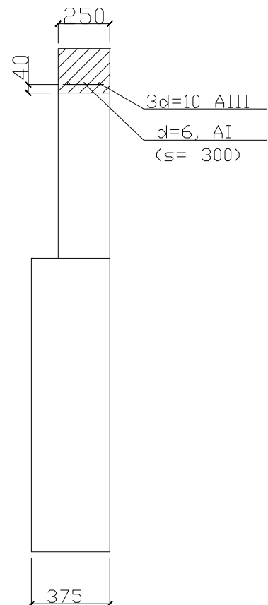
Lõige 1-1
