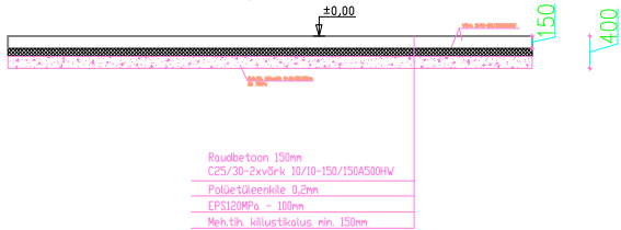
Lõige 1-1
