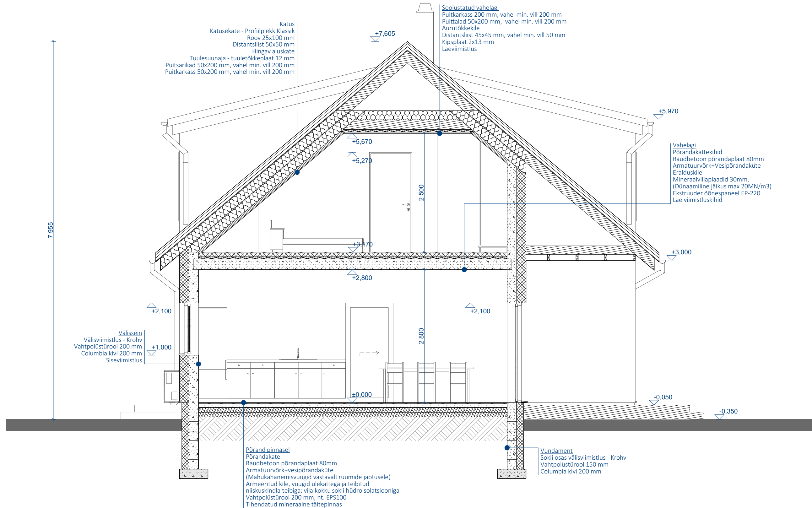
Joonis: LÕIGE 2-2
