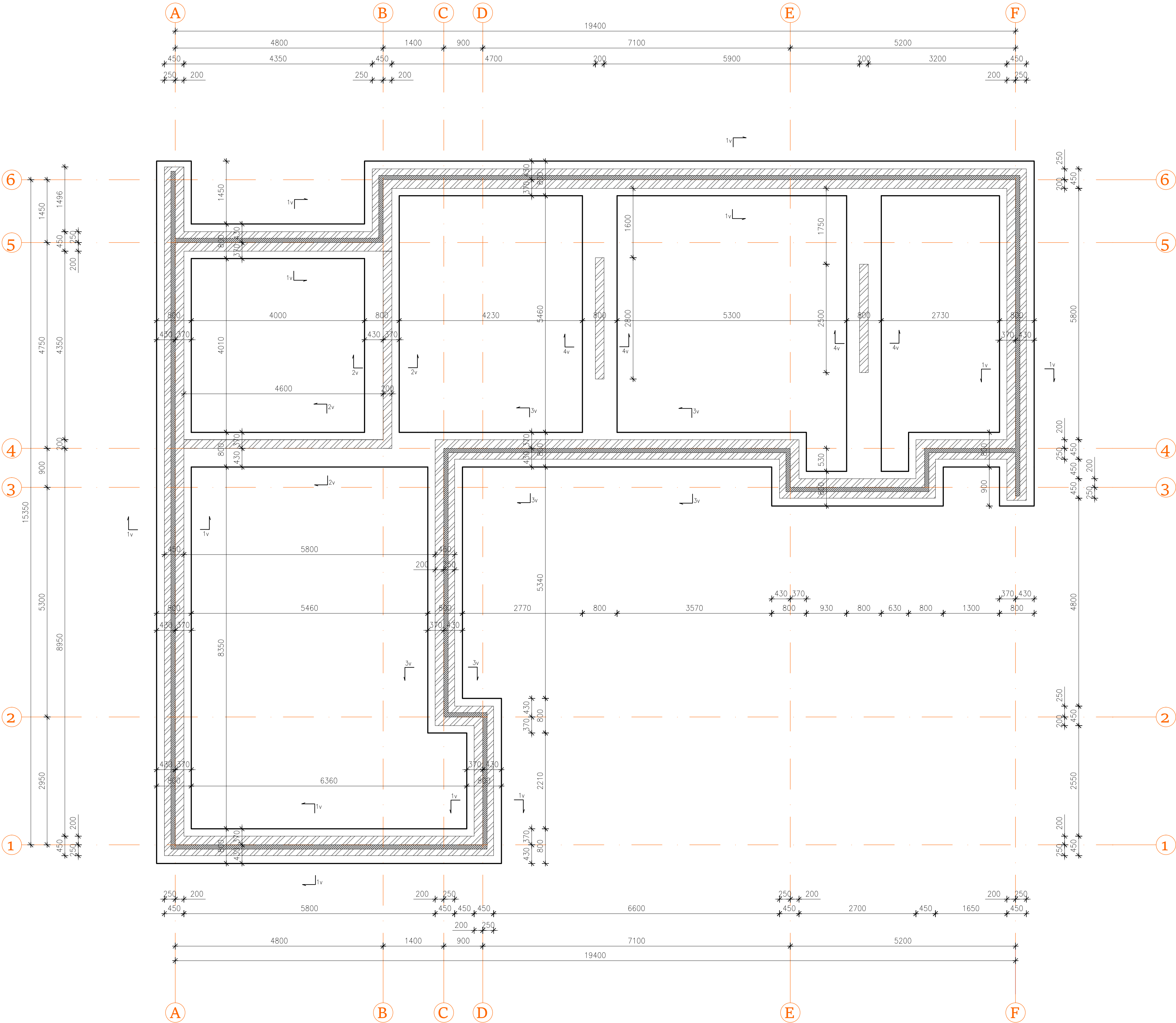
Vundamendi plaan M 1:50
