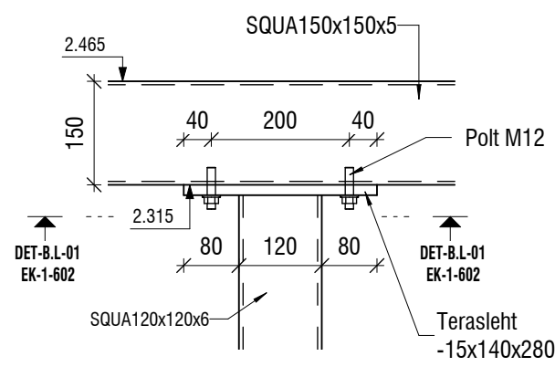
DET-B.L-01 EK-1-602/ 1:10
