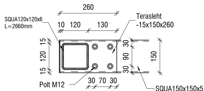
DET-A.L-01 EK-1-602/ 1:10
