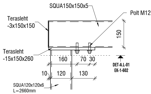
DET-A.L-01 EK-1-602/ 1:10
