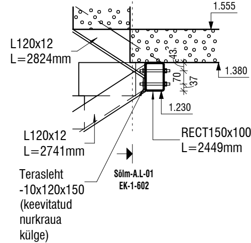
Sõlm-A EK-1-602/ 1:20
