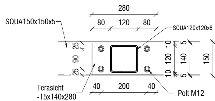
DET-B.L-01 EK-1-602/ 1:10
