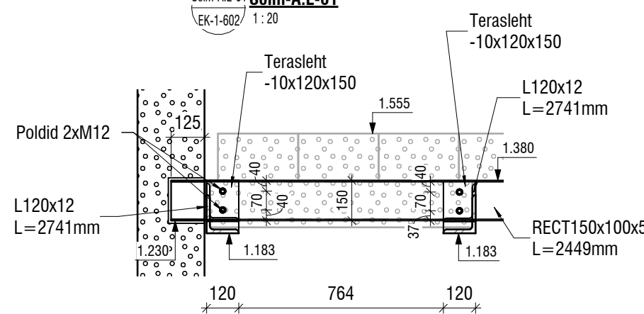
Sõlm-A.L-01 EK-1-602/ 1:20
