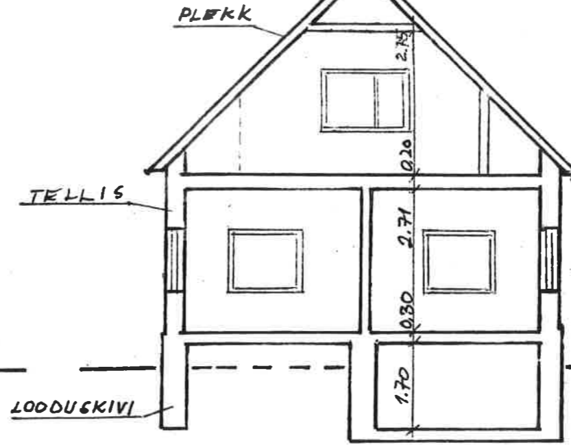
LÖIGE "A-A"
