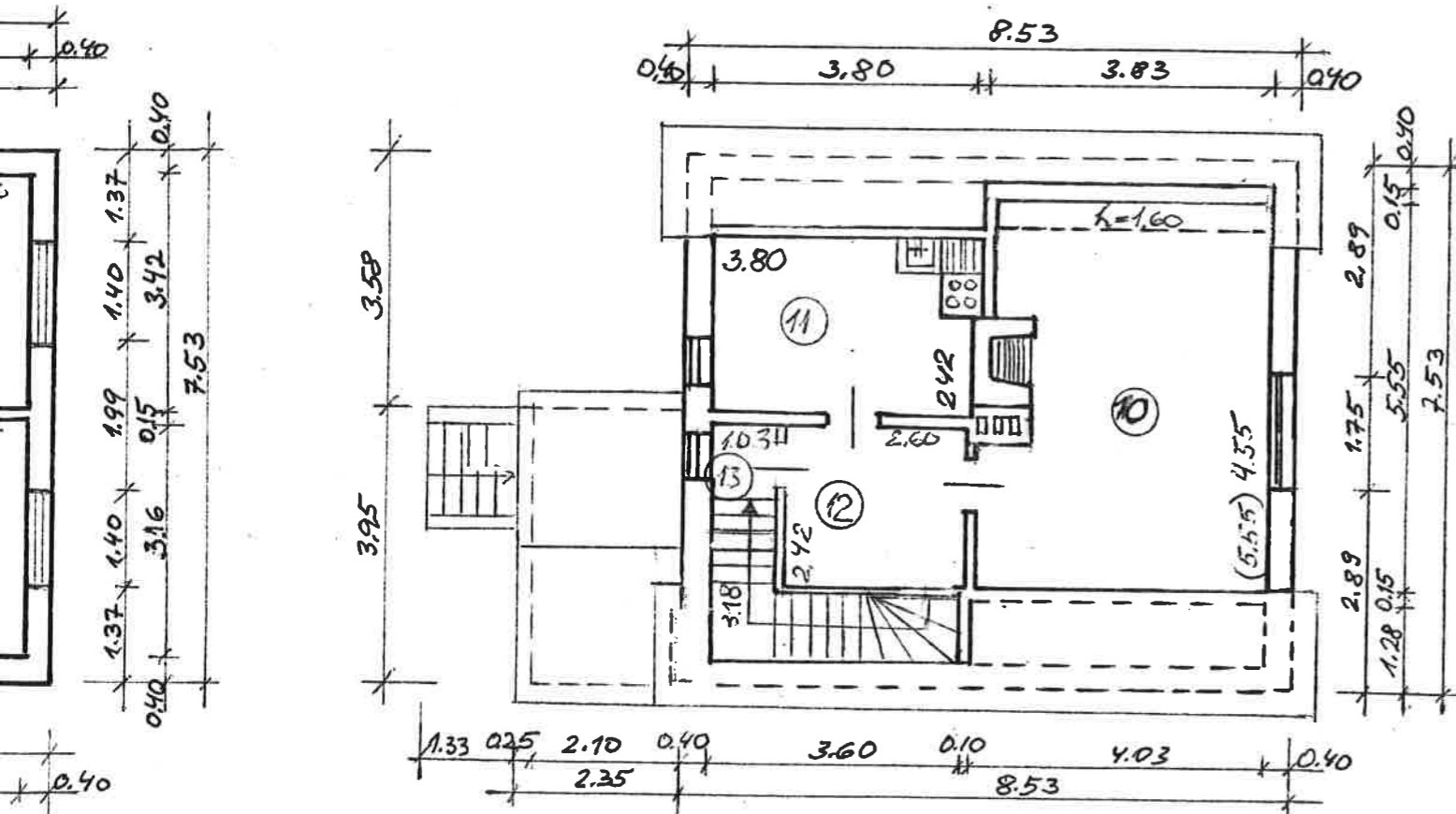
KATUSEKORRUSE PLAAN
